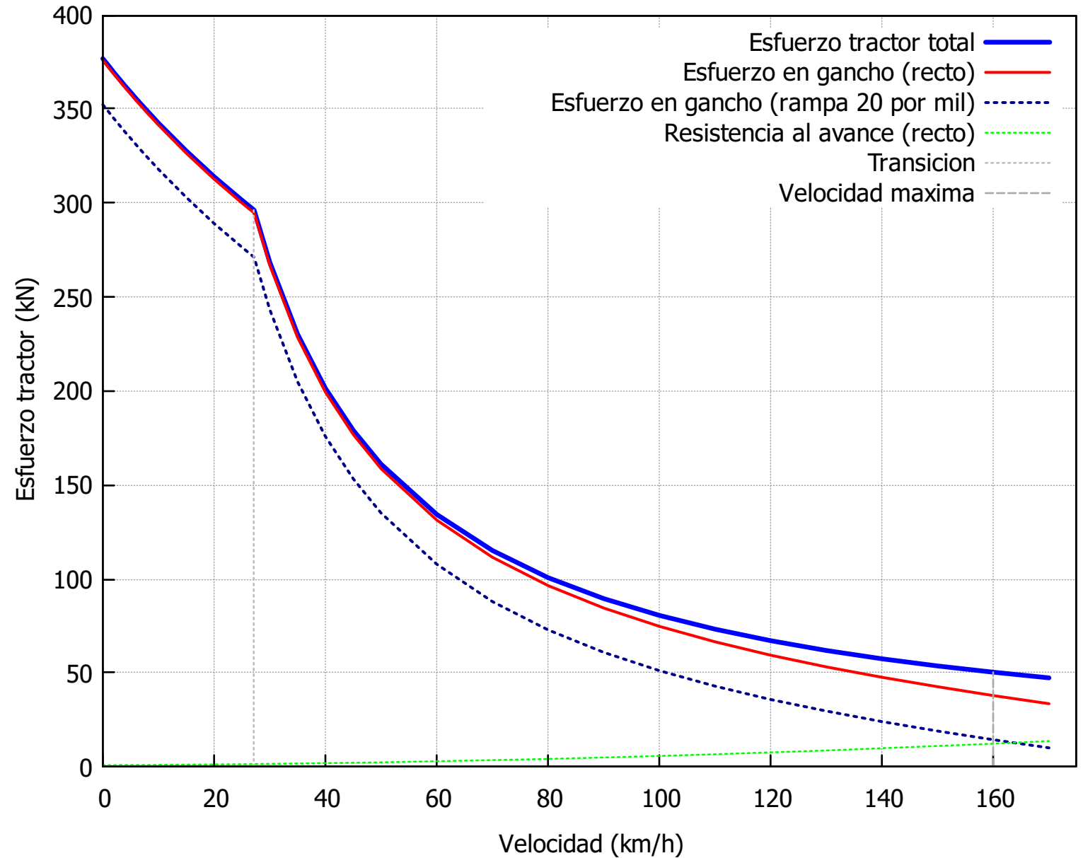
Curva de traccion - Renfe Serie 333.3
