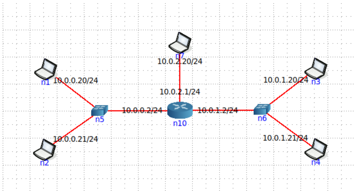
Topologia utilizada
