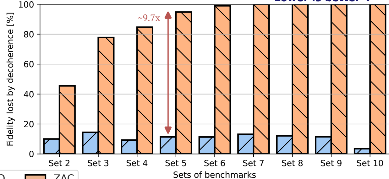
b) Decoherence error
