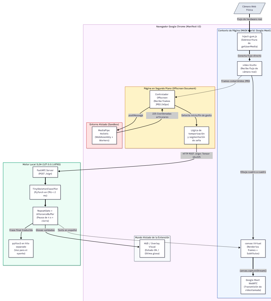
Figura 5.5: Arquitectura de integración en el navegador: intercepción de la cámara web, derivación de fotogramas al entorno aislado ( offscreen y sandbox ) y enlace con el motor local ILSA.
