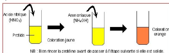
Réaction B
