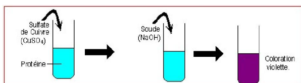
Réaction A
