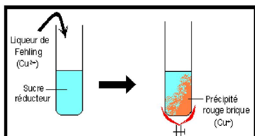
Réaction A
