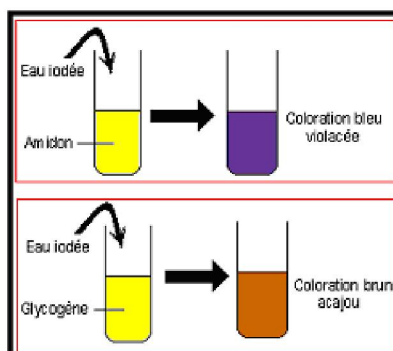
Réaction B
