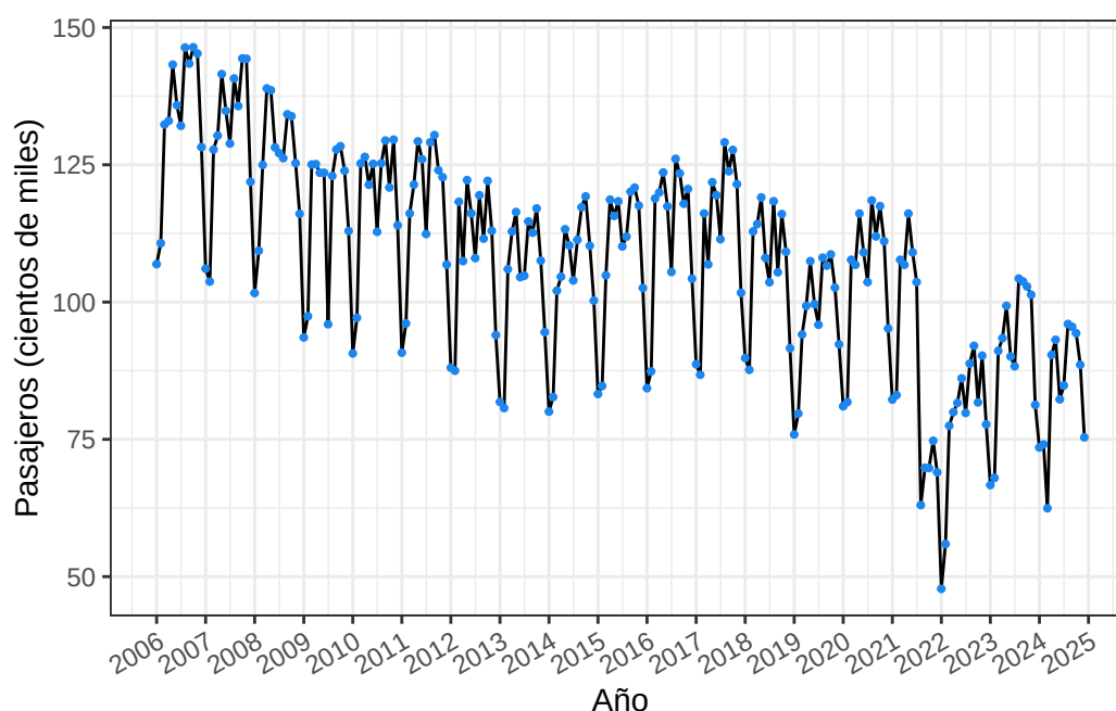
Figura 14: Pasajeros transportados por el sistema de Transporte Urbano de Pasajeros en la ciudad de Rosario. El período entre Marzo 2020 a Julio 2021 se reconstruyó utilizando el promedio de cada mes con los 3 años previos a Marzo 2020.
