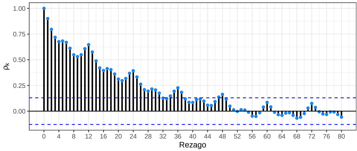
Figura 4: Función de autocorrelación muestral
