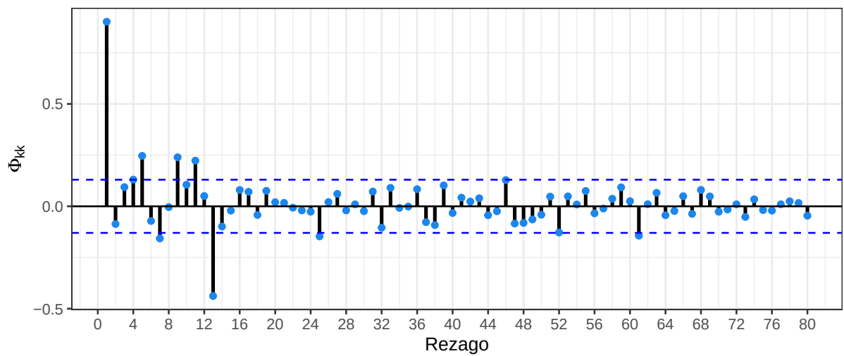
Figura 5: Función de autocorrelación parcial muestral
