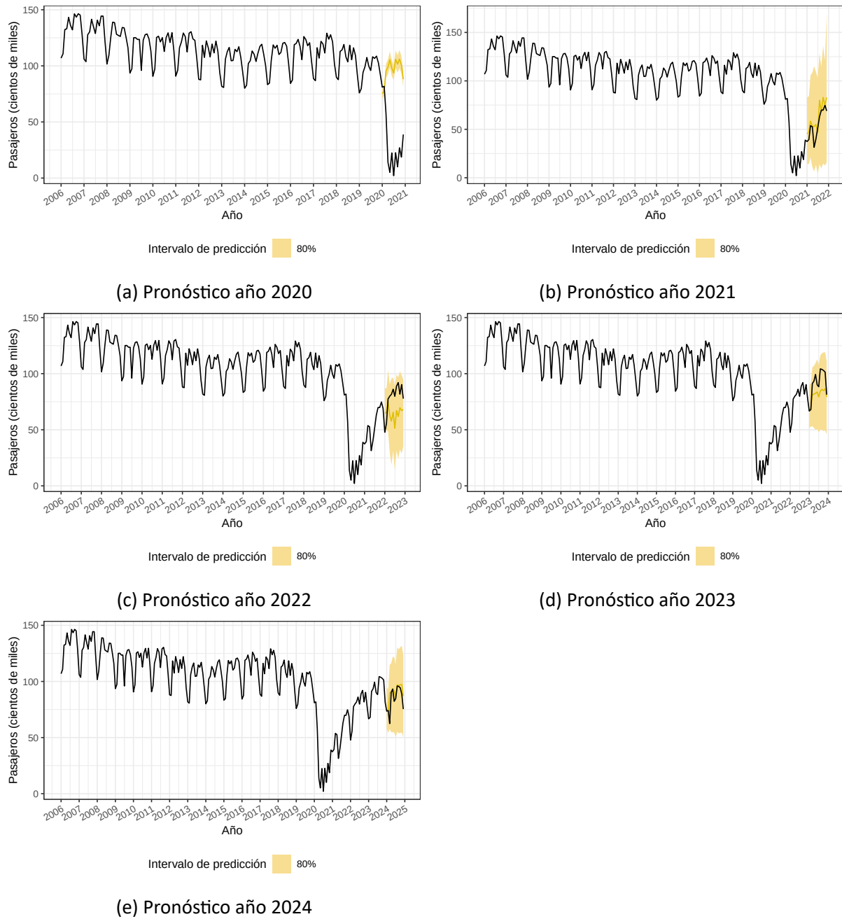
Figura 13: Pronósticos utilizando Ensemble
