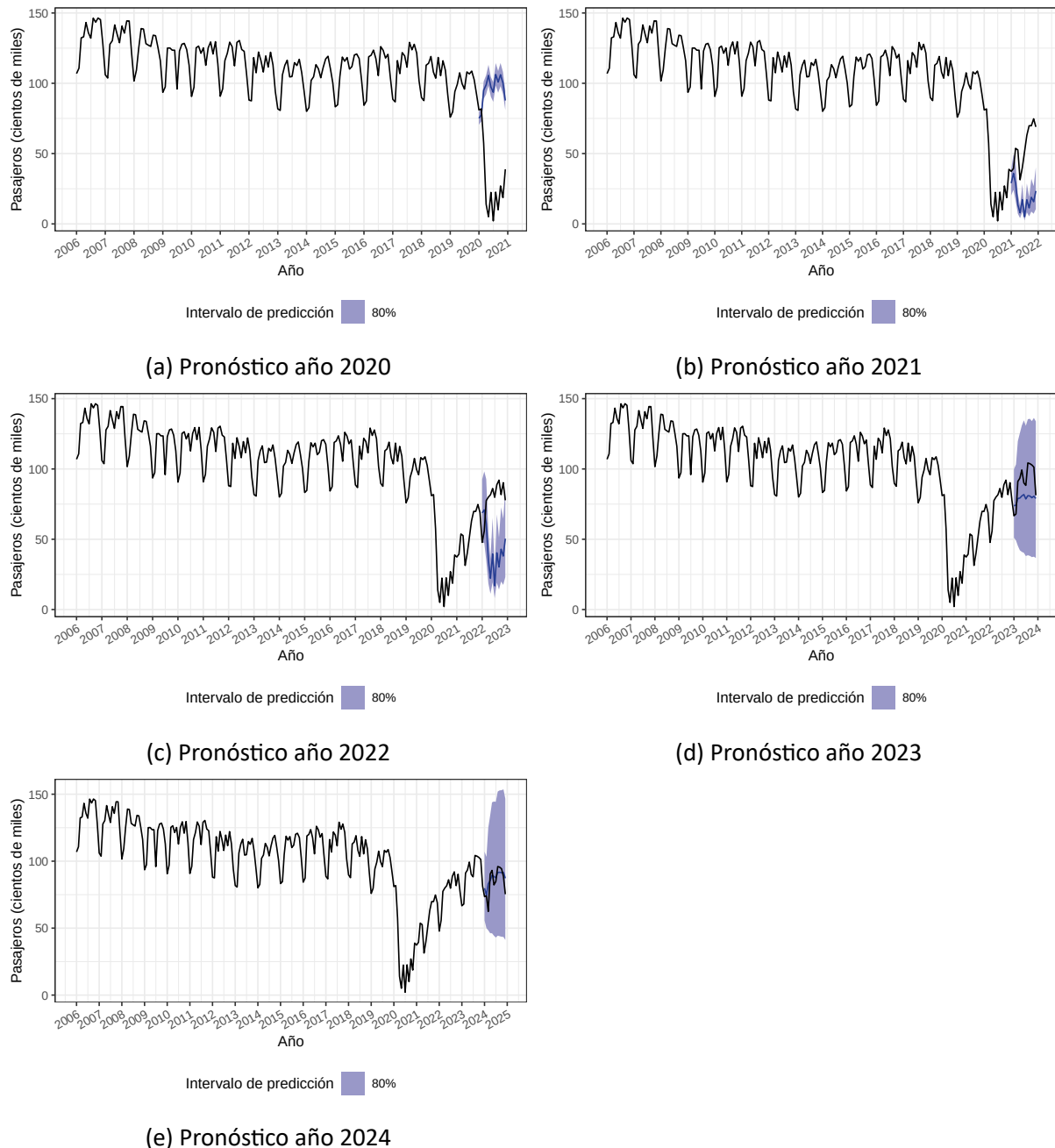
Figura 8: Pronósticos utilizando modelos ARIMA/SARIMA
