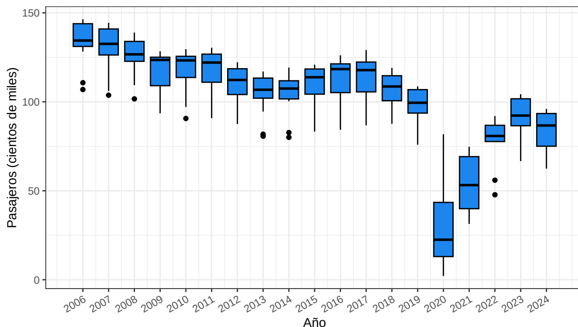
Figura 4: Distribución anual de pasajeros transportados por el sistema de Transporte Urbano de Pasajeros en la ciudad de Rosario.
