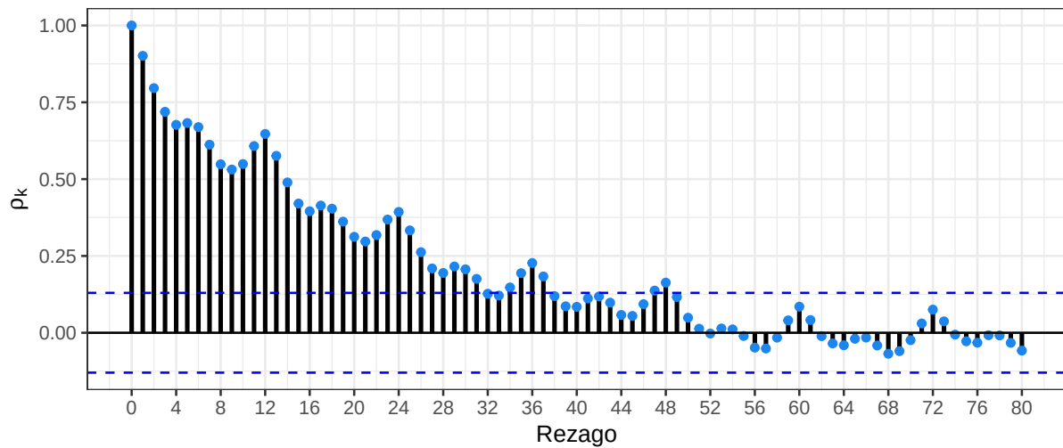
Figura 5: Función de autocorrelación muestral
