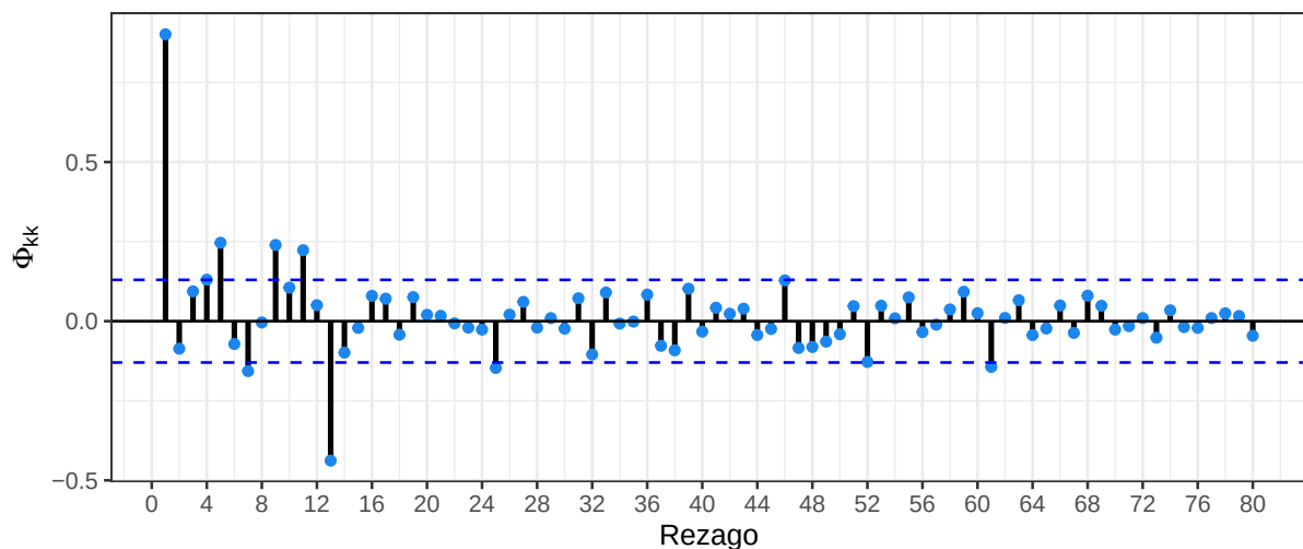
Figura 6: Función de autocorrelación parcial muestral
