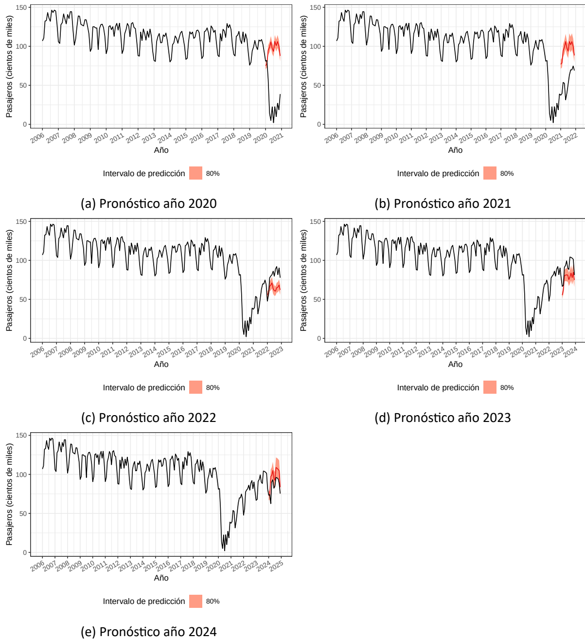
Figura 11: Pronósticos utilizando la estrategia 'establecer como faltante'
