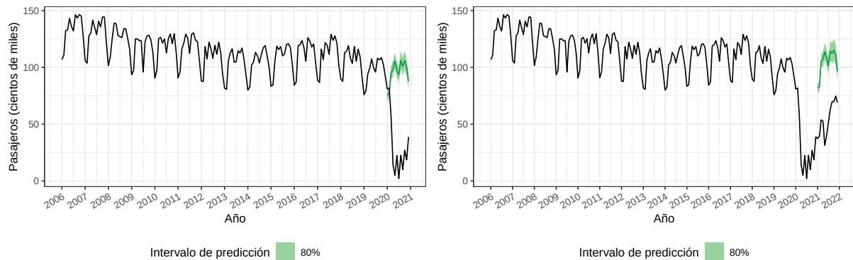
(a) Pronóstico año 2020
