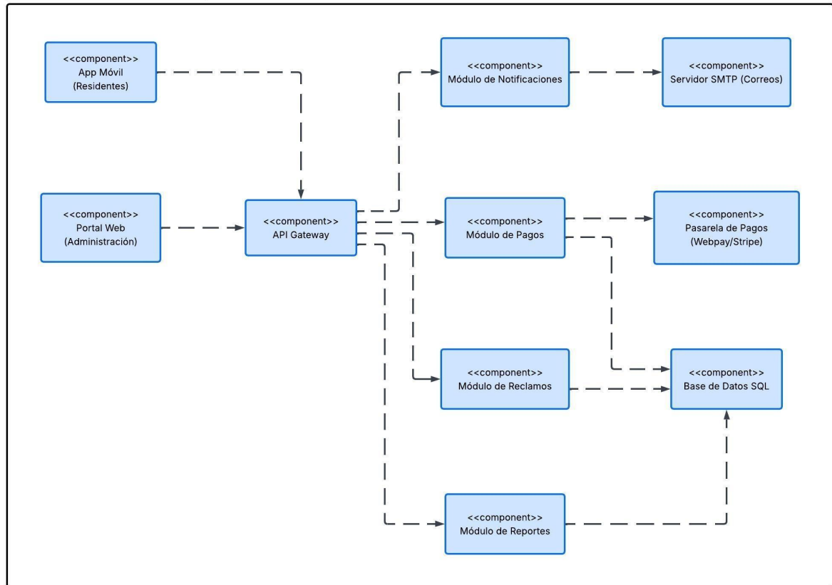
Diagrama de Componentes UML - El Mirador (Horizontal)
