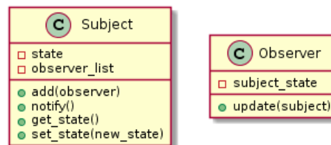
Figure 3: Le diagramme UML des classes Subject et Observer .
