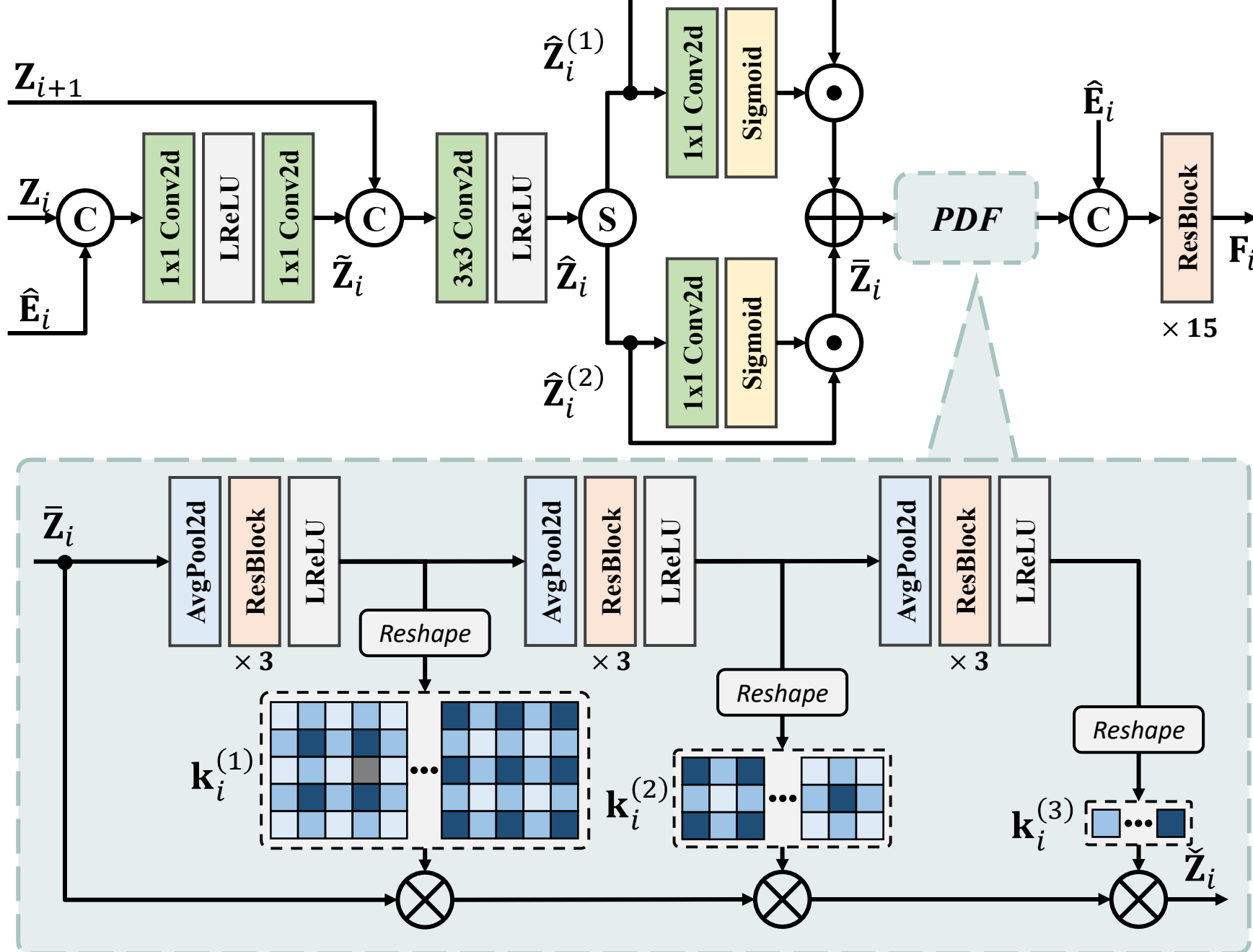
(d) Event-Guided Dynamic Feature Fusion (EGDFF) module
