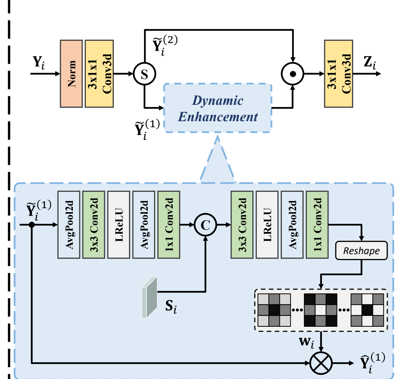
(c) Dynamic Spatial Enhancement (DSE) Module
