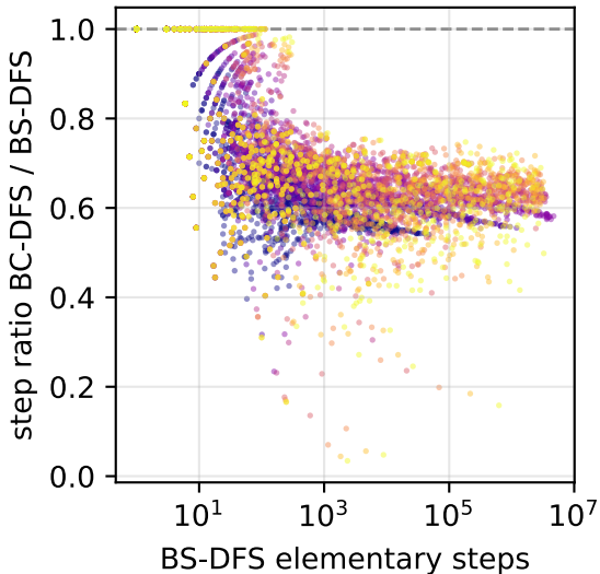
Erdős-Rényi
