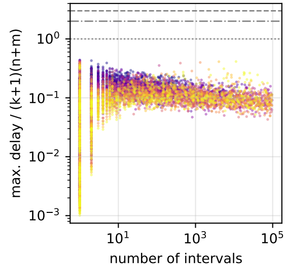
Erdős-Rényi
