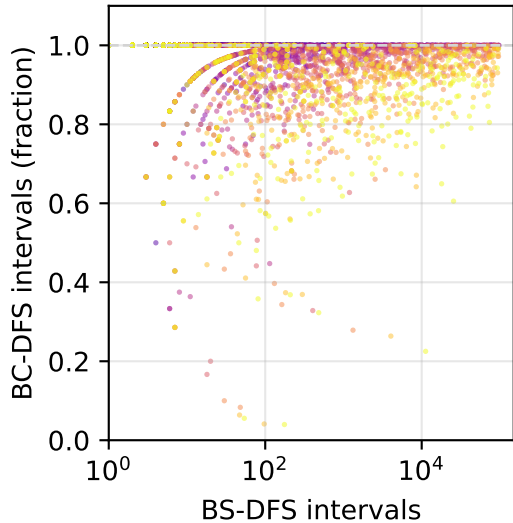
Erdős-Rényi
