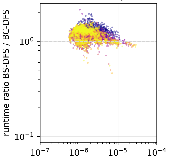
Barabási-Albert
