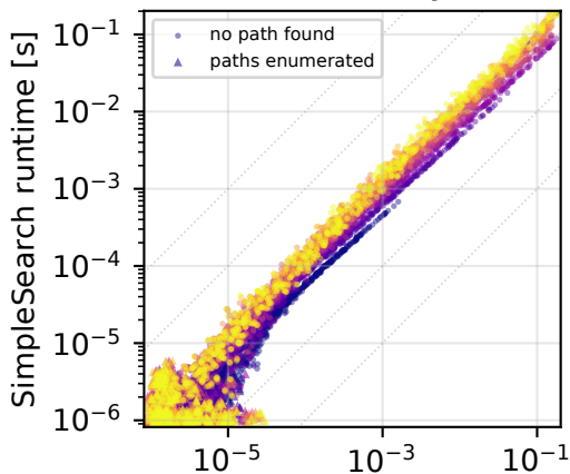
Erdős-Rényi
