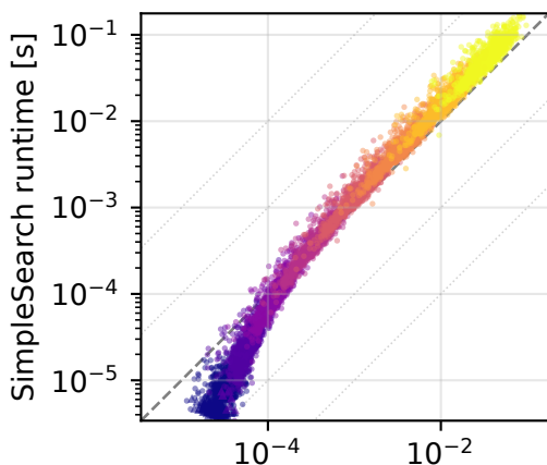
Barabási-Albert
