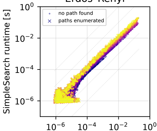
Erdős-Rényi
