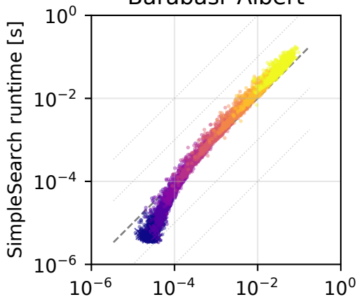
Barabási-Albert
