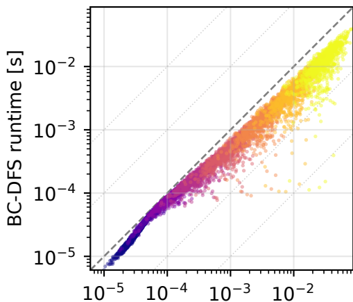
Barabási-Albert
