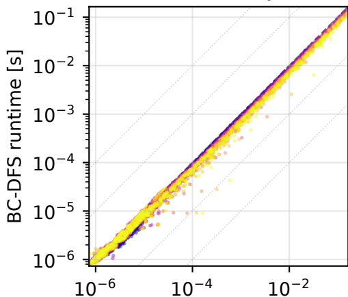
Erdős-Rényi
