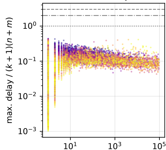
Barabási-Albert
