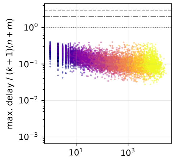
Barabási-Albert
