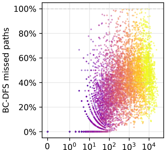
Barabási-Albert
