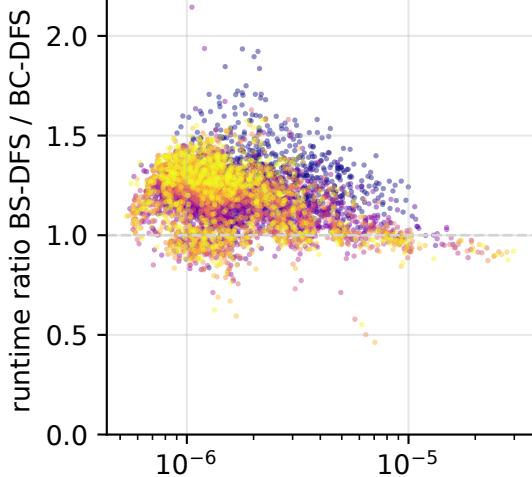
Barabási-Albert
