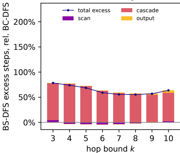
Barabási-Albert
