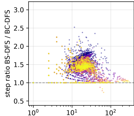
Erdős-Rényi
