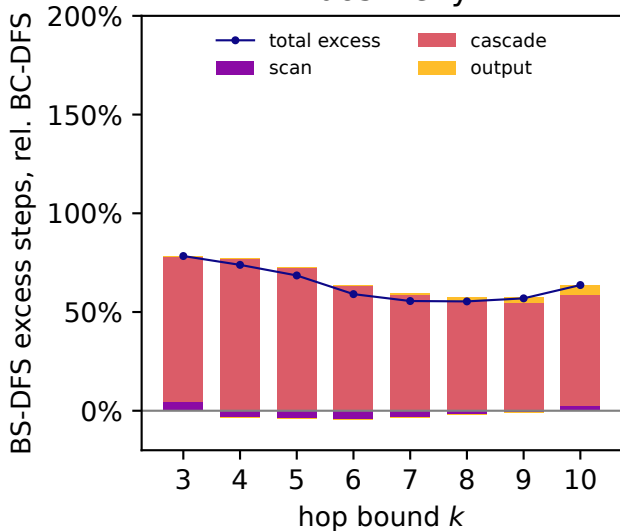
Erdős-Rényi
