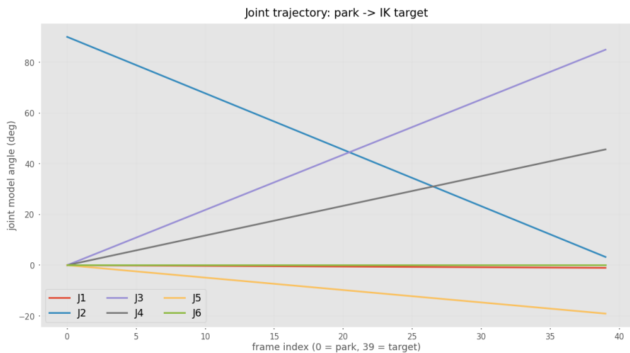
图 2: 目标运动过程中的关节角变化
