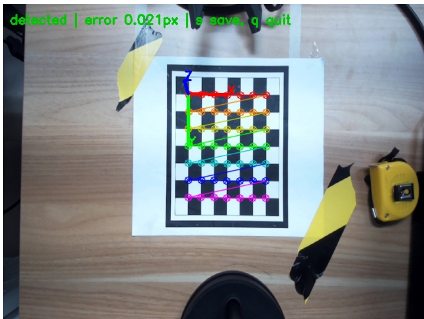
图 5: 棋盘格外参估计与坐标轴投影
