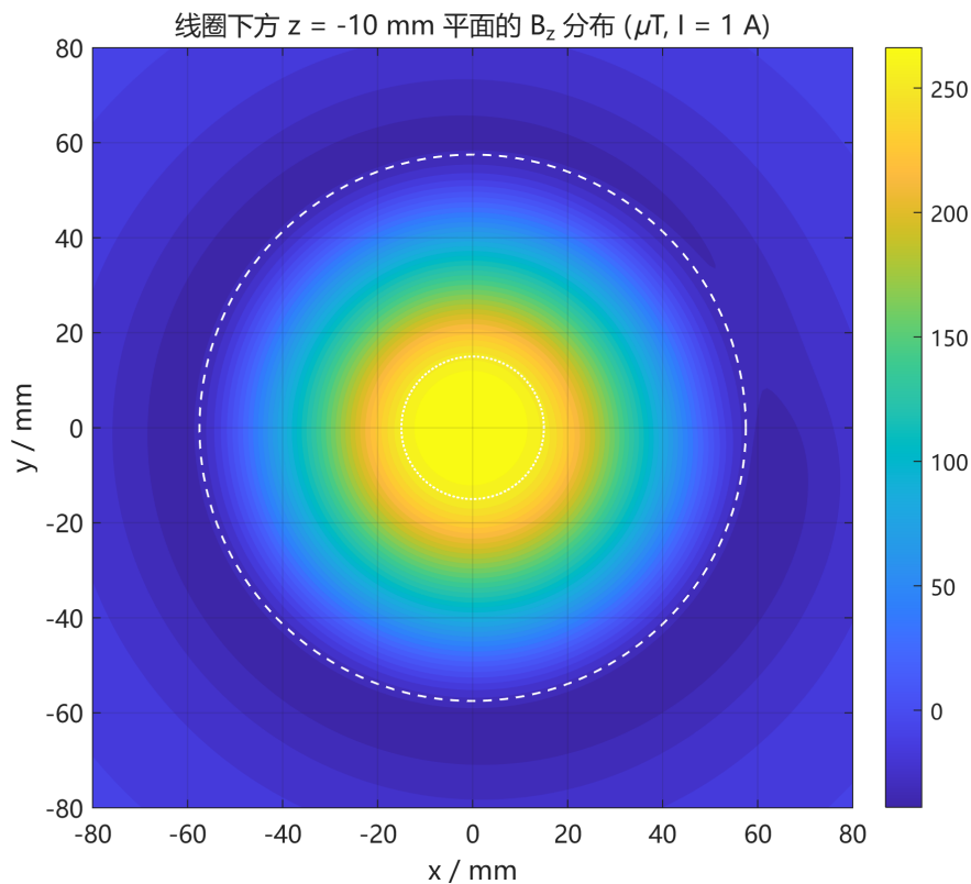
图 4: 线圈下方 z = -10 mm 平面的 B_z 分布 (1 A)
