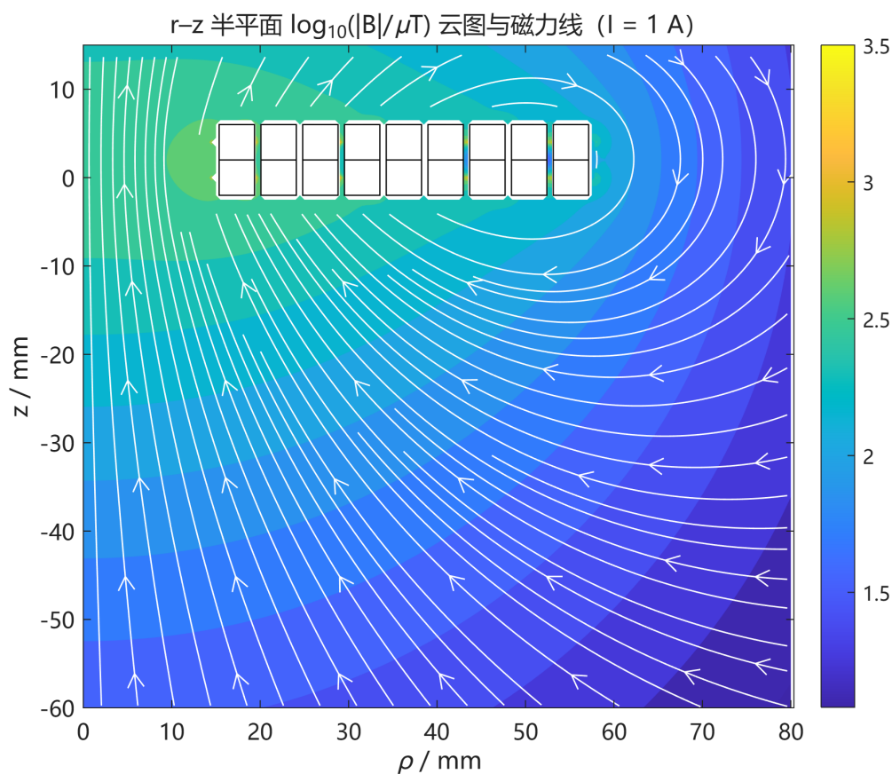
图 5: r - z 半平面 \log_{10}(|B|/\mu\text{T}) 云图与磁力线 (白色矩形为绕组截面, 1\text{ A} )
