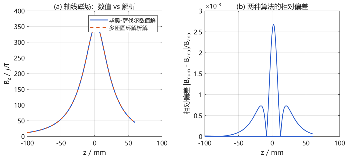
图 2: 轴线磁场: 数值解与多匝圆环解析解的对比 (a) 及相对偏差 (b)
