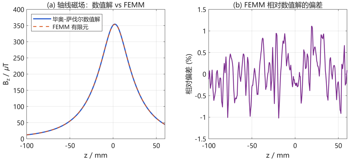
图 8: 轴线磁场: MATLAB 数值解与 FEMM 有限元解的对比 (a) 及相对偏差 (b)
