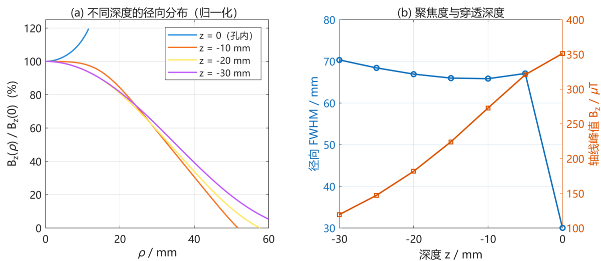
图 6: 聚焦性分析: (a) 不同深度的径向分布 (归一化); (b) 径向 FWHM 与轴线峰值随深度的变化
