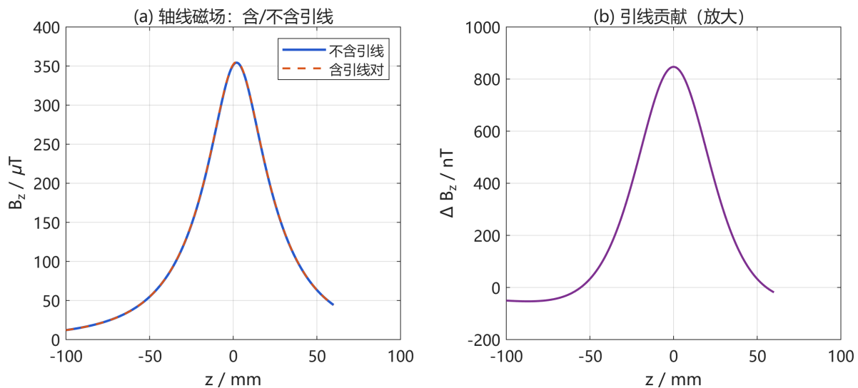
图 7: 引线影响：含/不含引线的轴线磁场（a）及引线贡献（b）
