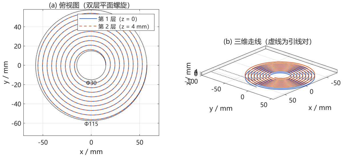
图 1: 圆形线圈计算模型: (a) 俯视图 (双层平面螺旋, 虚线圆为内外径); (b) 三维走线 (灰色虚线为引线对模型)
