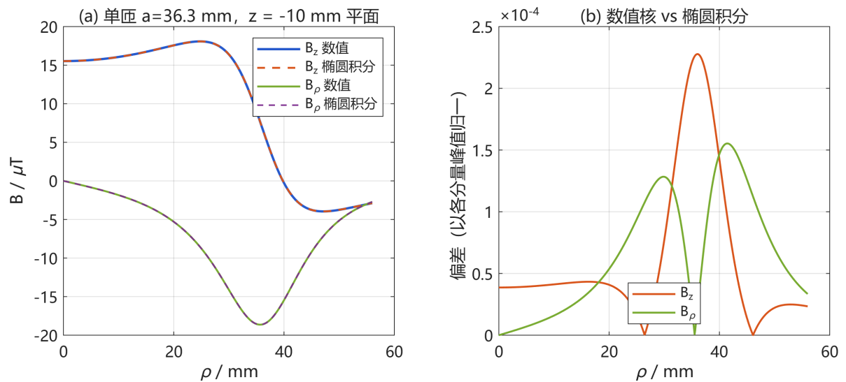
图 3: 单匝圆环离轴磁场: 直线单元数值解与椭圆积分精确解的对比 (a) 及峰值归一偏差 (b)
