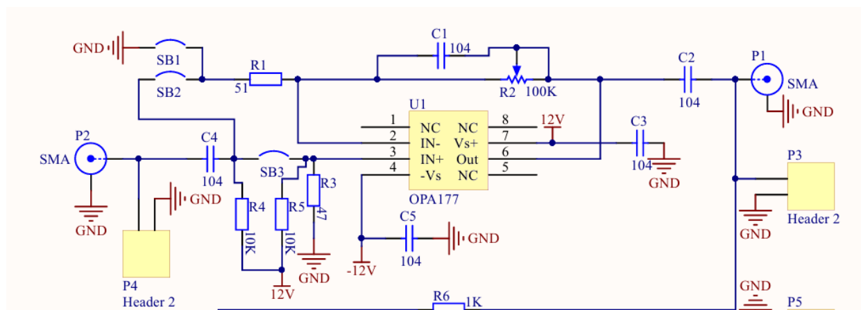
图 3: 后级放大模块原理示意
