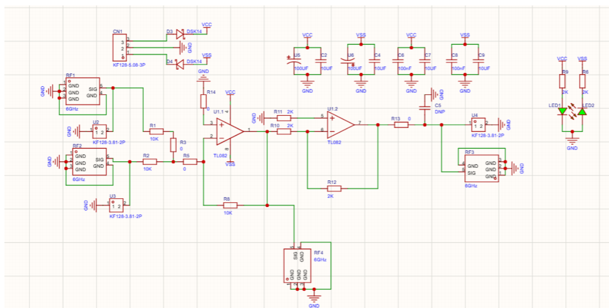
图 2: 独立加法器原理示意
