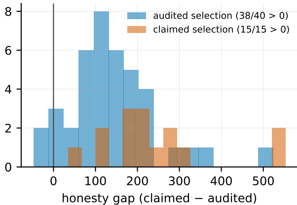
LunarLander-v3
