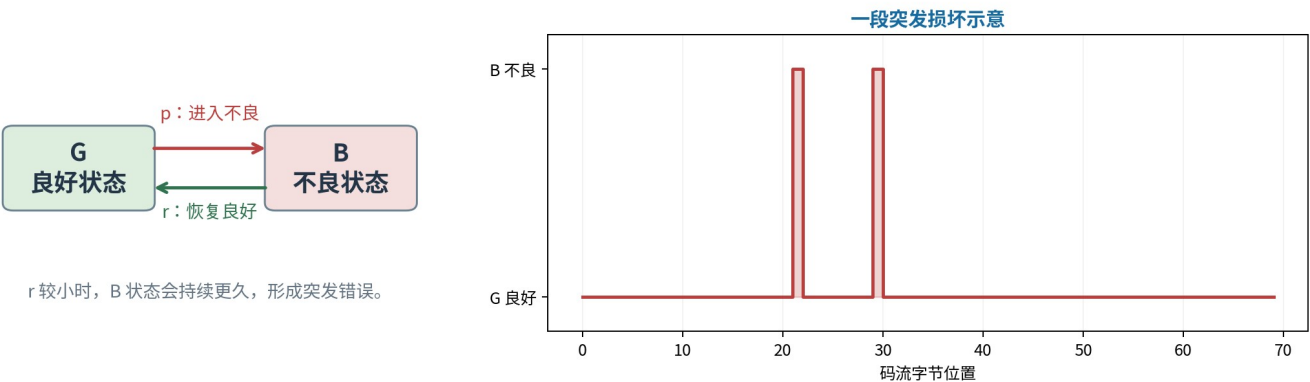
Gilbert-Elliott 二状态模型：用状态转移描述突发损坏
