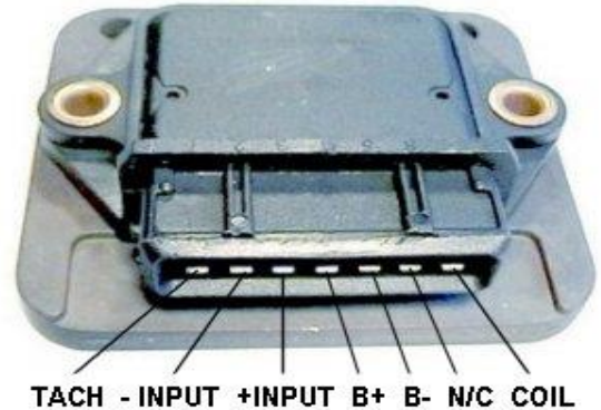
IGN MODULE TP900B MODULE VW KOMBIE
