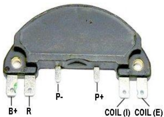
IGN MODULE J304
