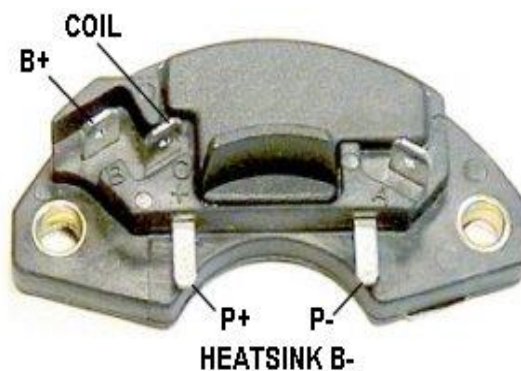
IGN MODULE IG-M008
