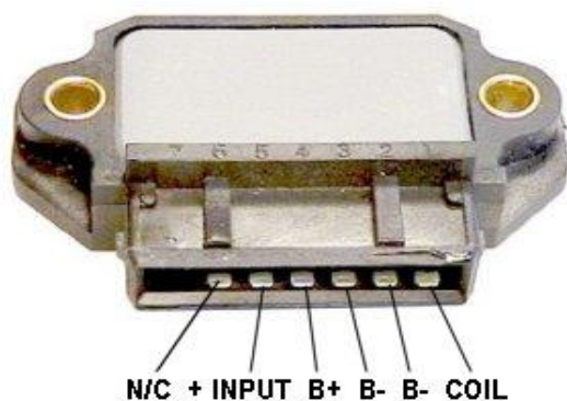
IGN MODULE IG-H006 6 PIN OPEL ASTRA/KADETT/MONZA
