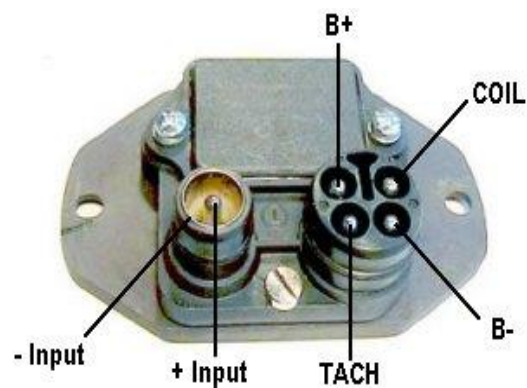
IGN MODULE TP1007B IGN MODULE MERC 1PIN & 4PIN
