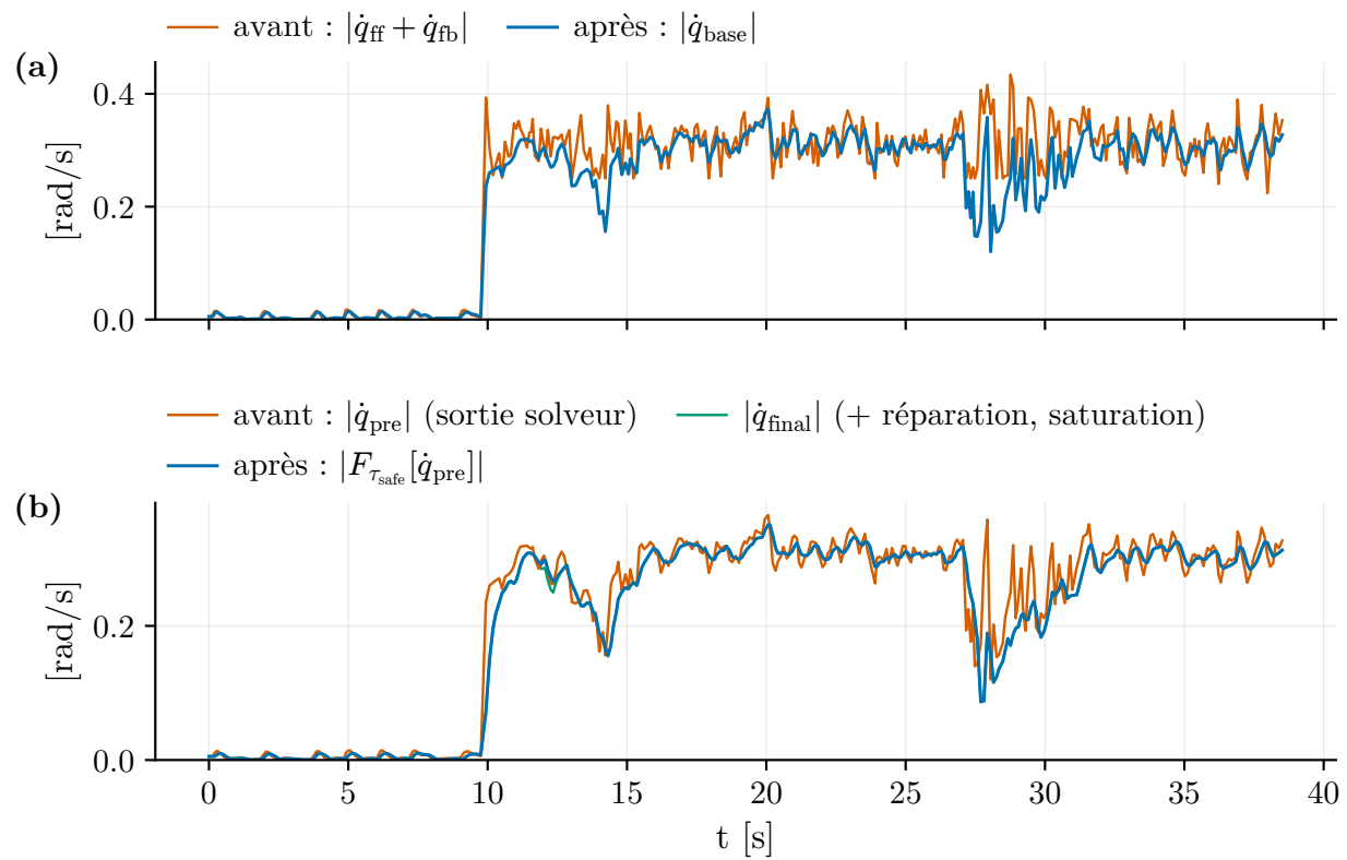
Figure 5.17 Norme de la vitesse sécurisée avant et après le filtre passe-bas de sortie ( \tau_{\text{safe}} = 0,2 s).
