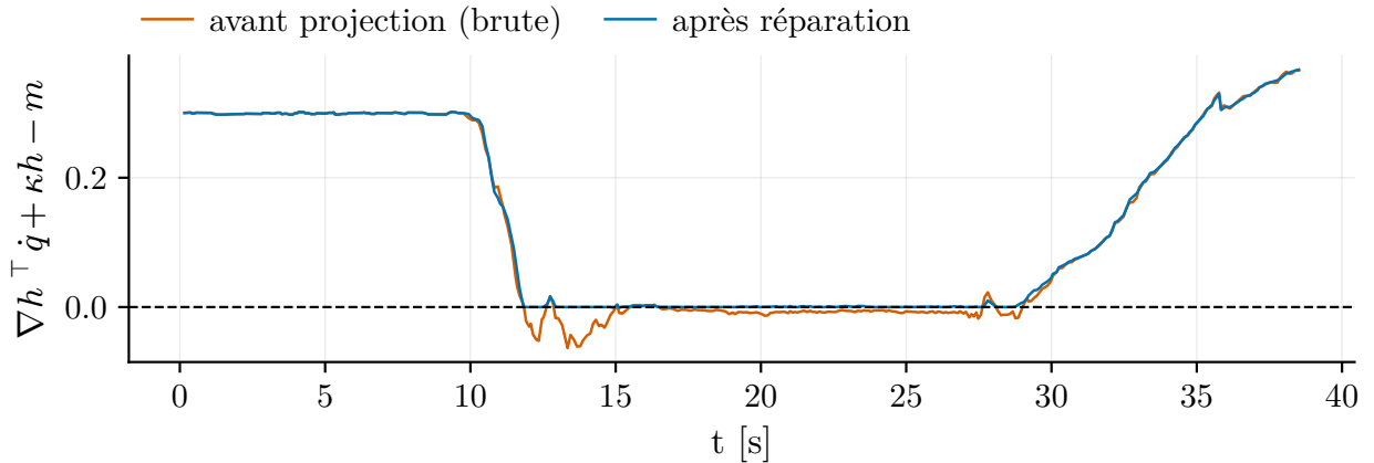
Figure 5.13 Contrainte de sécurité évaluée sur la vitesse nominale (avant projection) et sur la commande finale (après réparation). Les valeurs négatives de la courbe nominale correspondent aux violations qu'aurait commises la trajectoire générée sans filtre.
