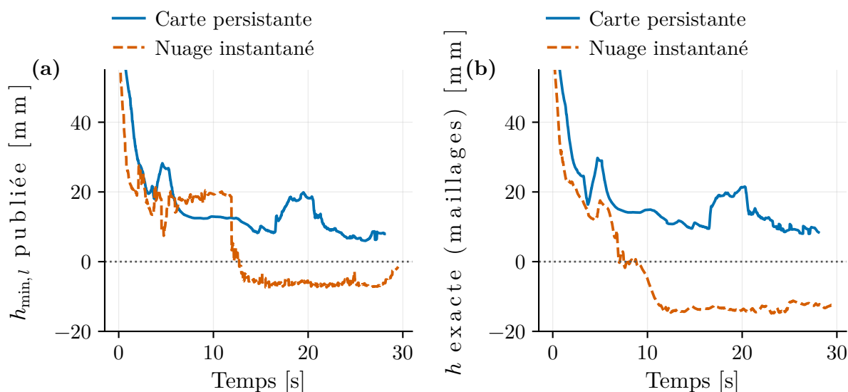
Figure 5.16 Ablation de la carte persistante sur le banc d'alimentation. (a) Barrière publiée en ligne; (b) barrière exacte recalculée hors ligne.
