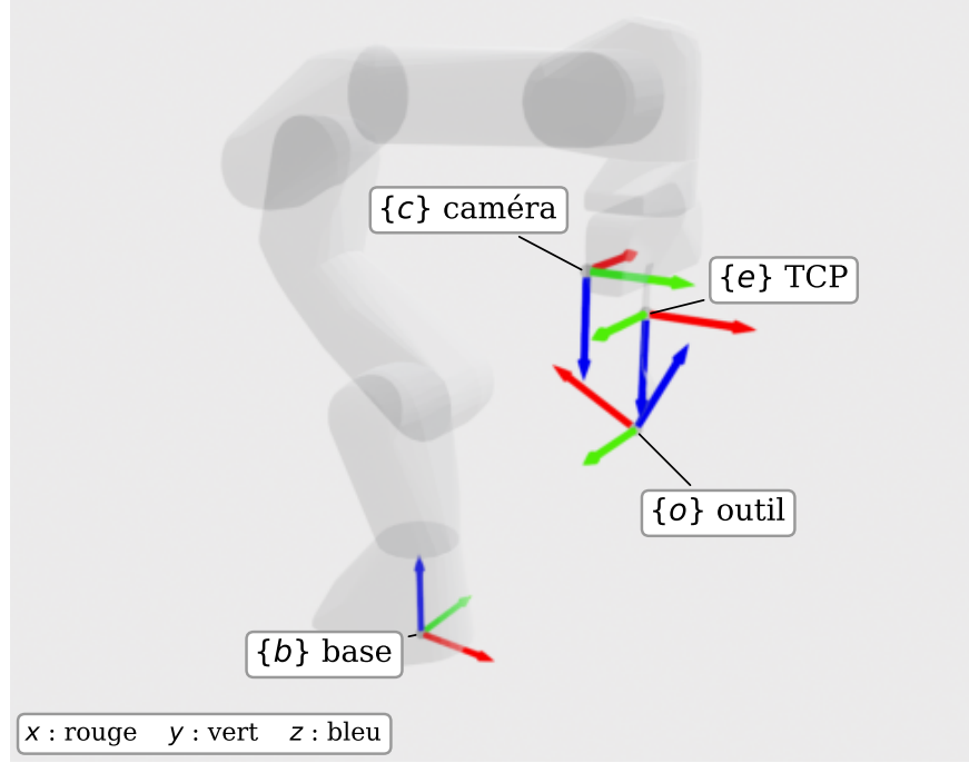
Figure 4.4 Représentation schématique des frames des différents repères utilisés
