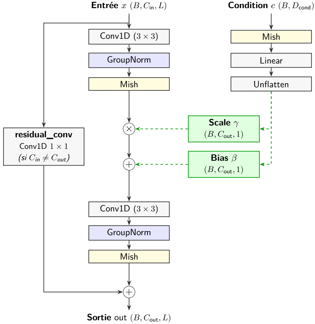
Figure 4.5 Architecture du module ConditionalResidualBlock1D avec un tracé orthogonal à angle droit unique vers les entrées latérales.
