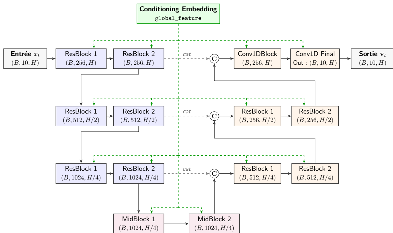
Figure 4.6 Architecture globale finale du ConditionalUnet1D au style épuré, corrigée de tout dépassement de tracé.
