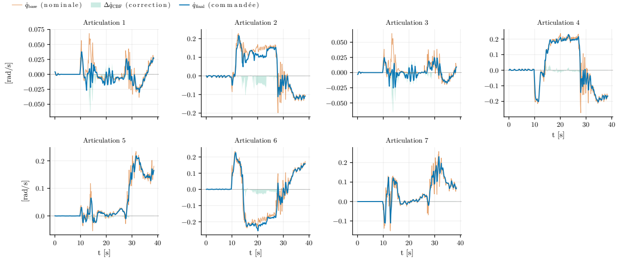
Figure 5.16 Action du filtre de sécurité : vitesse nominale et vitesse commandée superposées. Les surfaces teintées, restreintes aux cycles où le filtre intervient (projection ou réparation), distinguent le freinage de la poussée de récupération ; l'écart résiduel non teinté est l'effet du filtre passe-bas de sortie.
