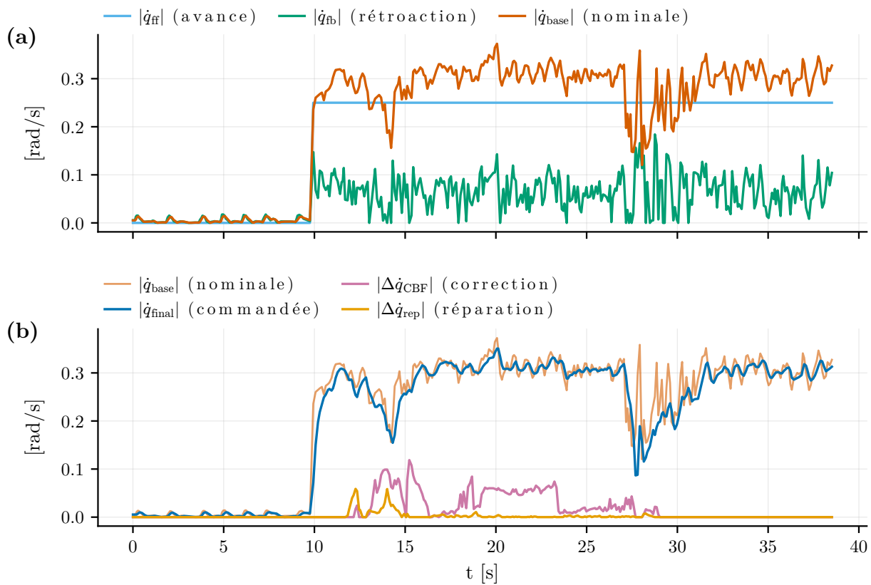
Figure 5.14 Décomposition des vitesses articulaires. (a) Construction de la vitesse nominale : feedforward retimé à norme constante \dot{q}_{ff} , correction de suivi \dot{q}_{fb} et vitesse nominale filtrée \dot{q}_{base} . (b) Action du filtre de sécurité : corrections de projection \Delta\dot{q}_{CBF} et de réparation \Delta\dot{q}_{rep} (reconstituée par rejeu du filtre de sortie), et vitesse commandée \dot{q}_{final} . Courbes lissées sur 0,25 s.
