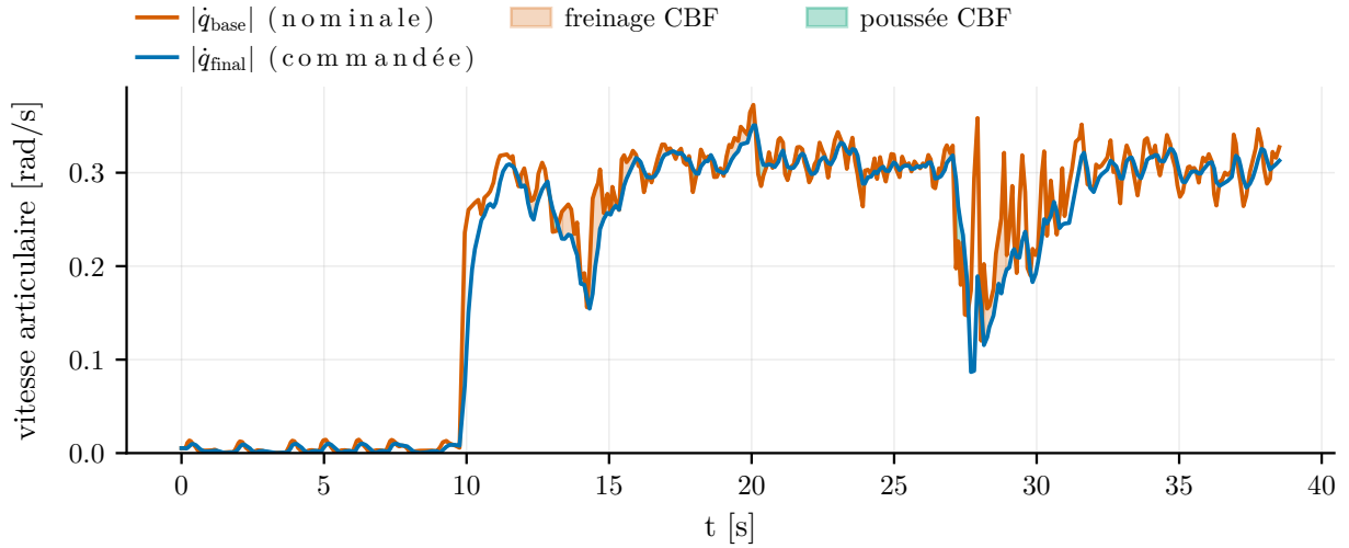
Figure 5.15 Action du filtre de sécurité : vitesse nominale et vitesse commandée superposées. Les surfaces teintées, restreintes aux cycles où le filtre intervient (projection ou réparation), distinguent le freinage de la poussée de récupération ; l'écart résiduel non teinté est l'effet du filtre passe-bas de sortie.
