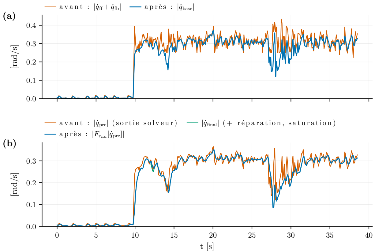
Figure 5.17 Norme de la vitesse sécurisée avant et après le filtre passe-bas de sortie ( \tau_{safe} = 0,2 s).
