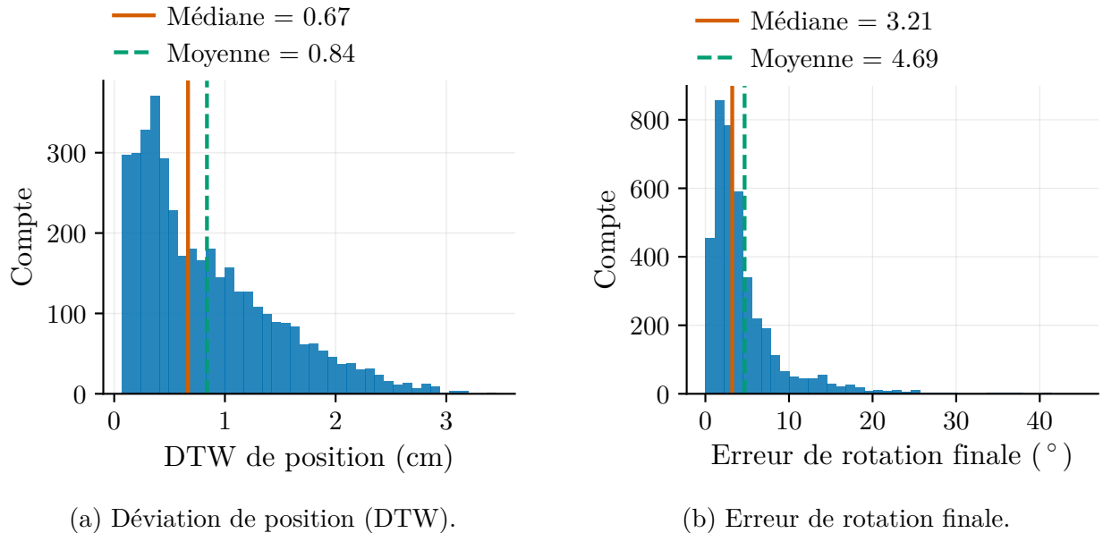
Figure 5.6 Fidélité du planificateur nominal aux démonstrations expertes sur le jeu de validation. (a) Distribution de la déviation de position (DTW) ; (b) distribution de l'erreur de rotation finale à l'effecteur.
