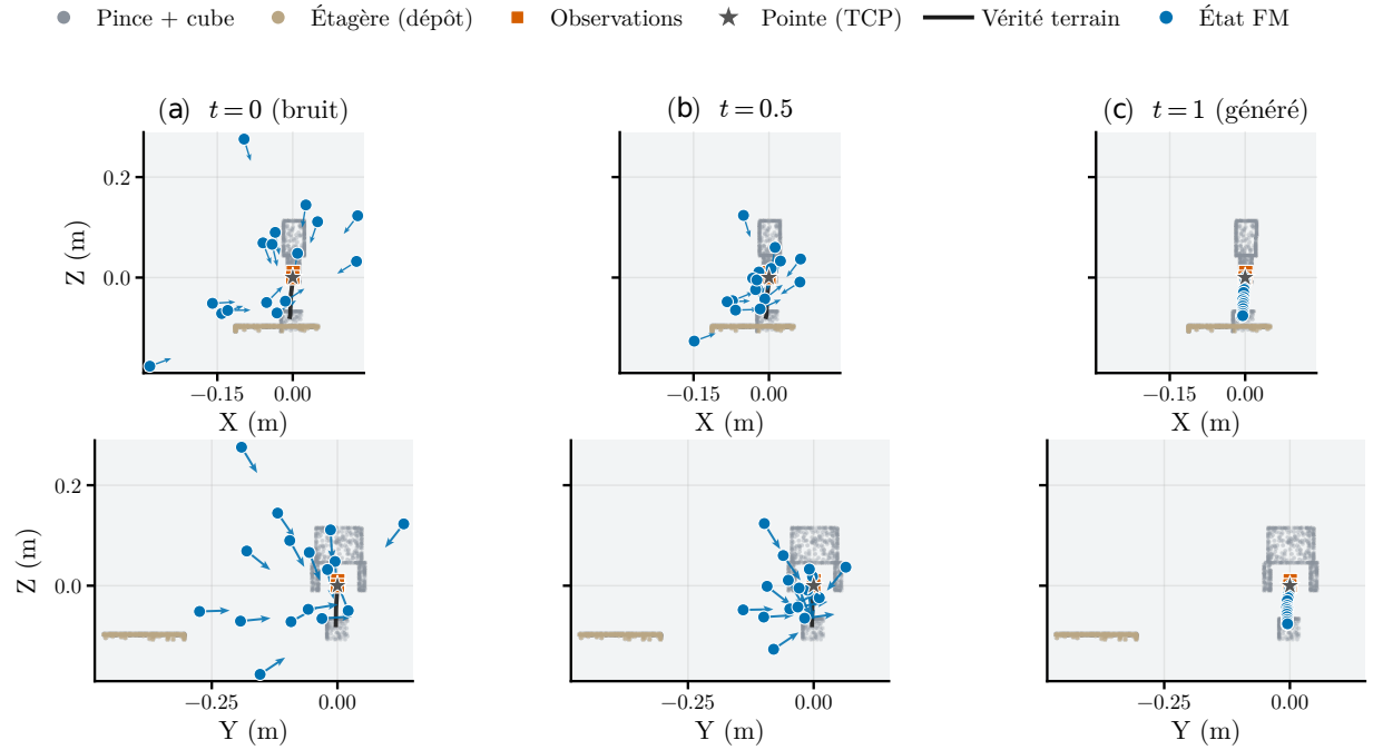
Figure I.12 Intégration du flot pour une scène de la tâche de saisie et dépôt : segment X_t à t = 0 (bruit), t = 0,5 et t = 1 (génééré).
