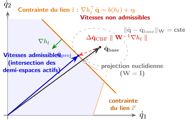
Figure 4.7 Interprétation géométrique, dans un plan de l'espace des vitesses articulaires, de la projection de sécurité (4.12) : la vitesse nominale filtrée \dot{\mathbf{q}}_{\text{base}} est projetée sur l'intersection des demi-espaces actifs \nabla h_l^T \dot{\mathbf{q}} \geq b(h_l) + \eta_l , dont les normales \nabla h_l pointent vers l'intérieur. La solution \dot{\mathbf{q}}_{\text{proj}} est le point où le plus petit ellipsoïde de niveau de la métrique de tâche \mathbf{W} centré sur \dot{\mathbf{q}}_{\text{base}} touche la frontière : la correction \Delta \dot{\mathbf{q}}_{\text{CBF}} suit la direction \mathbf{W}^{-1} \nabla h_l et non la normale, et s'écarte ainsi de la projection euclidienne ( \mathbf{W} = \mathbf{I} , point creux), en déplaçant le moins possible le lien contrôlé.
