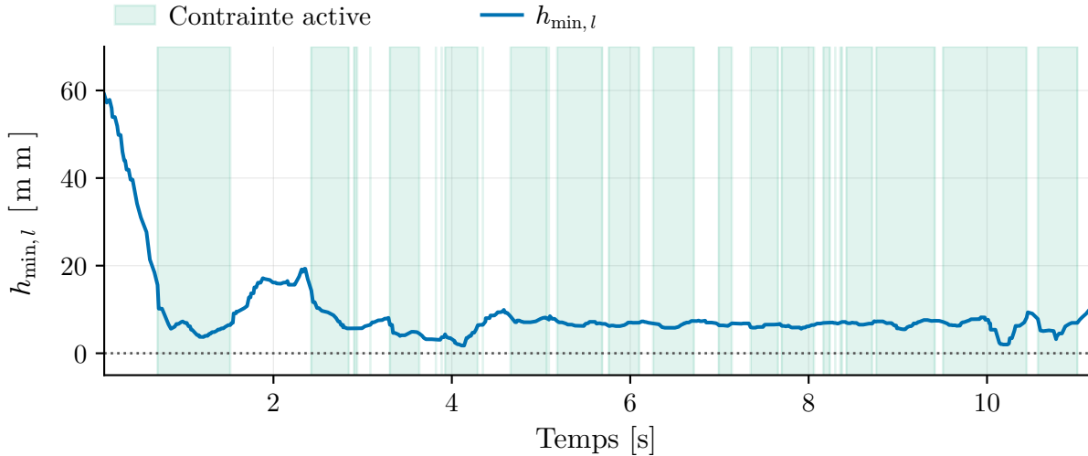
Figure 5.8 Évolution de la barrière h_{\text{min},l} pour une tâche en présence d’obstacles ; les bandes ombrées indiquent les cycles où la vitesse nominale filtrée \dot{\mathbf{q}}_{\text{base}} viole la contrainte de la ligne critique.
