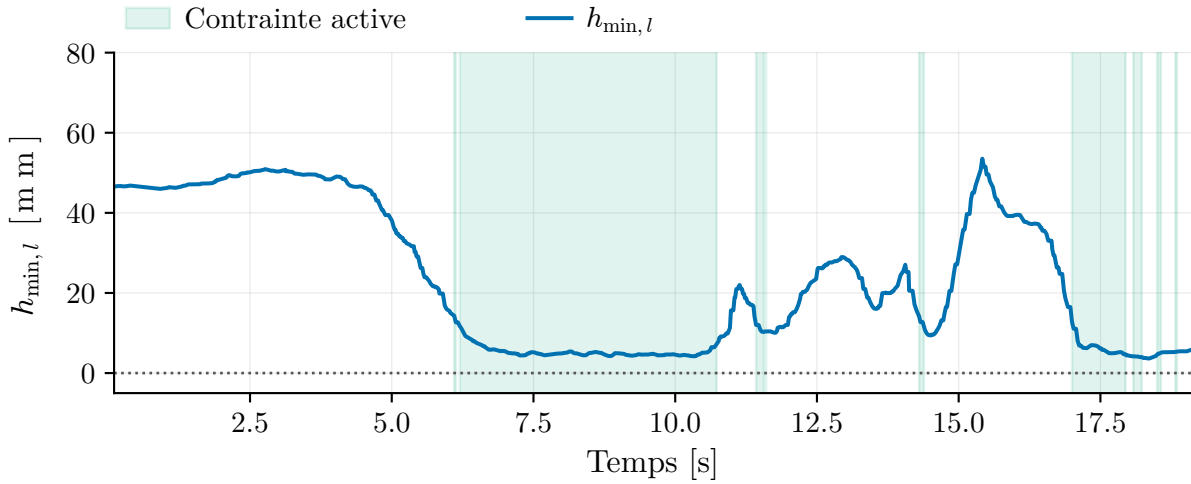
Figure 5.12 Essai représentatif de la tâche de saisie et dépôt en présence du prisme statique : évolution de la barrière h_{\min,l} . Les bandes ombrées marquent les cycles où la contrainte de la ligne critique, évaluée sur la vitesse nominale filtrée \dot{\mathbf{q}}_{\text{base}} , est violée.
