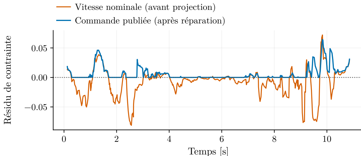
Figure 5.7 Contrainte de sécurité évaluée sur la vitesse nominale (avant projection) et sur la commande finale (après réparation). Les valeurs négatives de la courbe nominale correspondent aux violations qu’aurait commises la trajectoire générée sans filtre.
