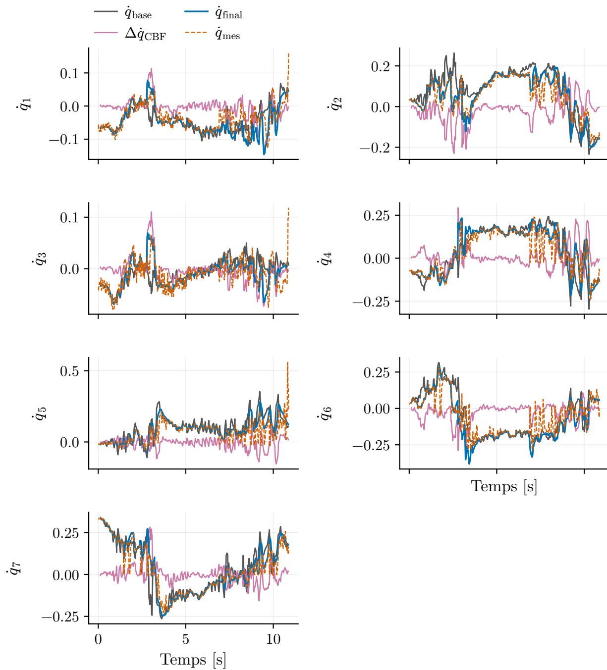
Figure I.15 Vitesse nominale, correction de projection, vitesse commandée et vitesse mesurée pour chacune des sept articulations.
