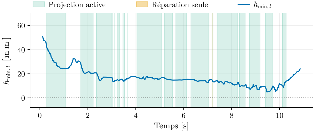
Figure 5.6 Évolution de la barrière h_{\min,l} pour une tâche en présence d'obstacles ; les bandes vertes indiquent les cycles où la projection corrige la vitesse, les bandes jaunes ceux où seule la réparation intervient.
