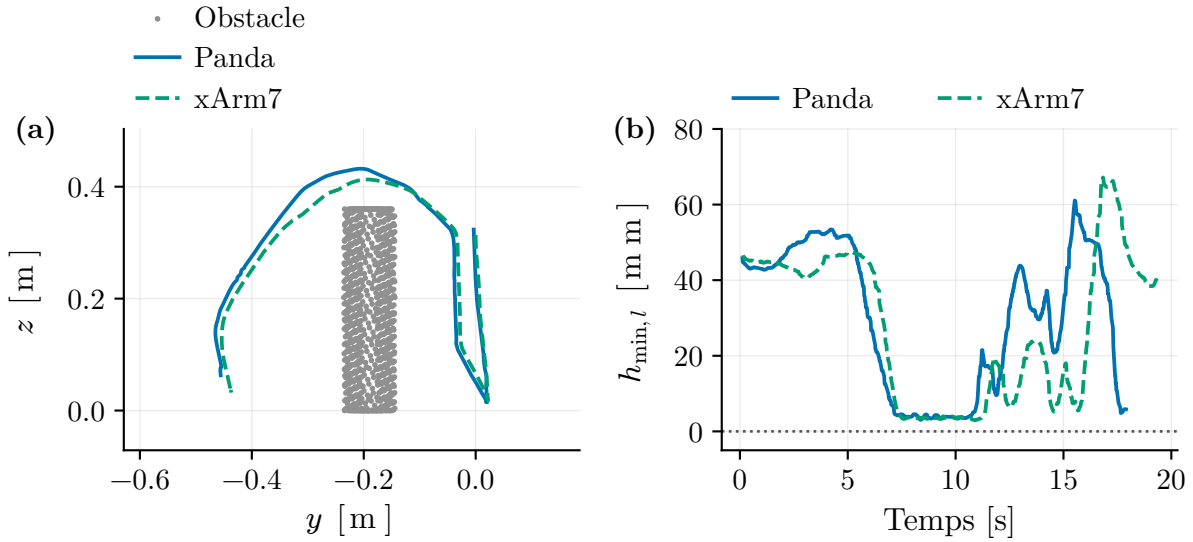
Figure 5.11 Panda et xArm7 sur une même graine du scénario à prisme statique. (a) Trajectoire de la pointe de l'outil dans le plan yz , superposée au nuage d'obstacles ; (b) barrière h_{\min, t} au cours de l'essai.
