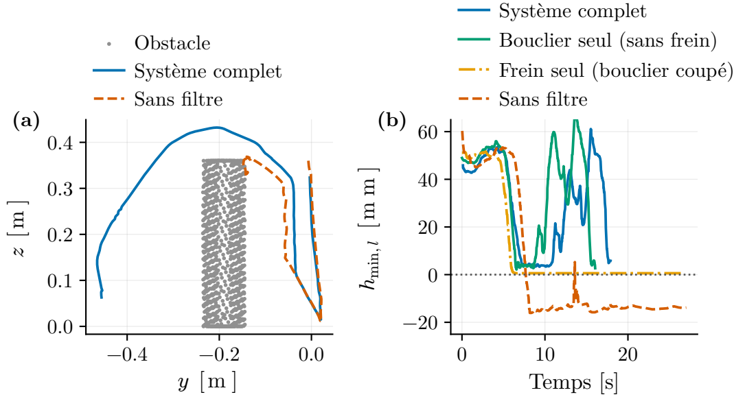
Figure 5.5 Comparaison des quatre conditions sur une même graine du banc de saisie et dépôt (prisme statique). (a) Trajectoire de la pointe de l'outil dans le plan yz , superposée au nuage d'obstacles ; (b) barrière h_{\min,l} au cours de l'essai.
