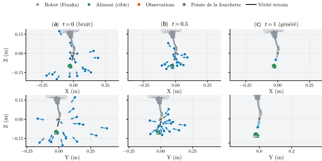
Figure I.12 Intégration du flot pour une scène de la tâche d'alimentation : segment X_t à t=0 (bruit), t=0,5 et t=1 (généré), dans les plans XZ (haut) et YZ (bas).
