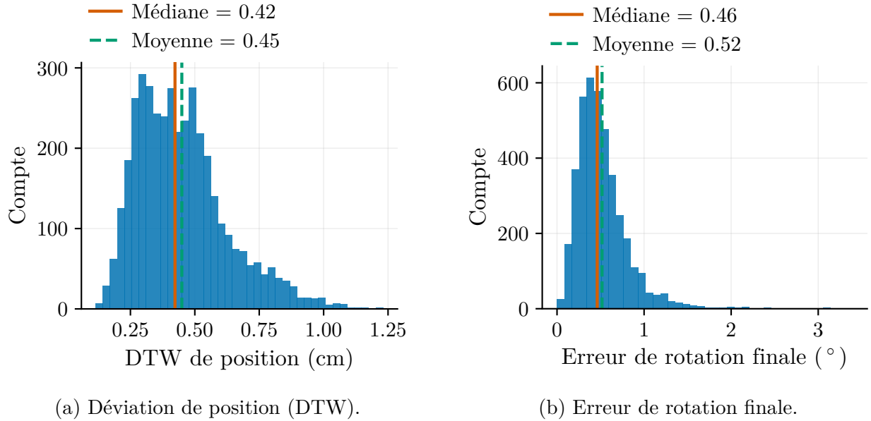
Figure I.17 Fidélité du planificateur nominal aux démonstrations expertes pour la tâche de saisie et dépôt. (a) Distribution de la déviation de position (DTW); (b) distribution de l'erreur de rotation finale à l'effecteur.
