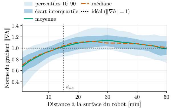
(b) Norme du gradient (propriété eikonale).
