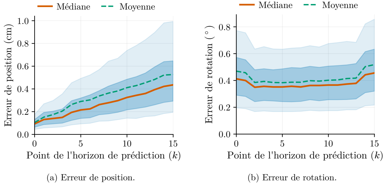
Figure I.18 Erreur de prédiction en fonction du point k de l'horizon pour la tâche de saisie et dépôt. (a) Erreur de position; (b) erreur de rotation. Bandes : percentiles 10 à 90 et écart interquartile.
