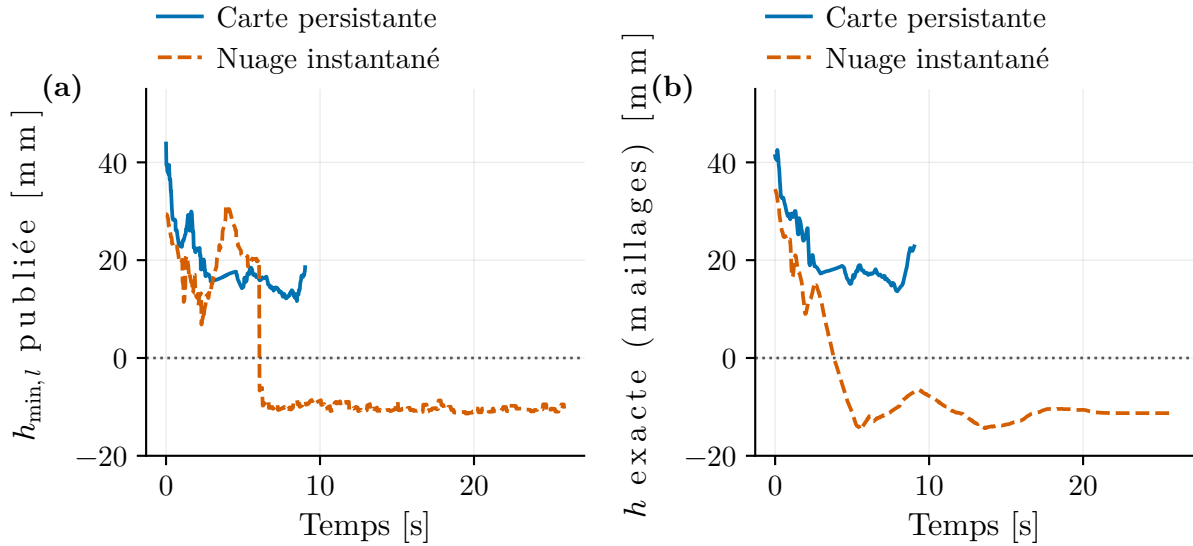
Figure 5.9 Ablation de la carte persistante sur une même graine du banc d'alimentation. (a) Barrière publiée par le nœud ; (b) barrière exacte recalculée hors ligne sur les maillages. Sans mémoire spatiale, la barrière exacte franchit zéro près de trois secondes avant que la barrière publiée ne le signale.
