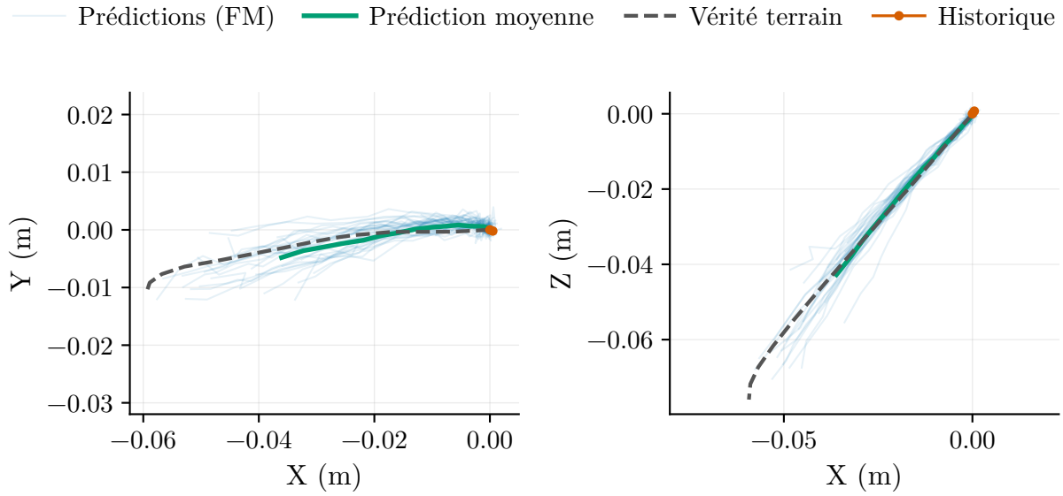
Figure I.11 Générations multiples du planificateur pour une même observation, superposées à la vérité terrain. (a) Plan XY ; (b) plan XZ .
