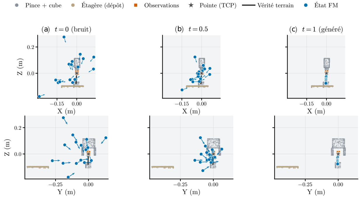
Figure I.20 Intégration du flot pour une scène de la tâche de saisie et dépôt : segment X_t à t=0 (bruit), t=0,5 et t=1 (généré).
