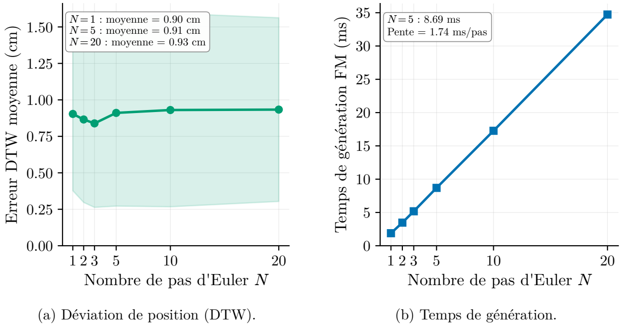
Figure I.4 Qualité et coût de la génération selon le nombre de pas d'Euler N . (a) La déviation DTW moyenne demeure pratiquement constante sur toute la plage, son minimum se situant à N = 3 ; (b) le temps de génération croît linéairement, à pente constante.
