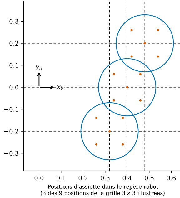
Figure 4.5 Grille d'échantillonnage des cibles et des assiettes dans le repère \mathcal{F}_b (vue de dessus, seules trois des neuf positions de la grille 3 × 3 illustrées).
