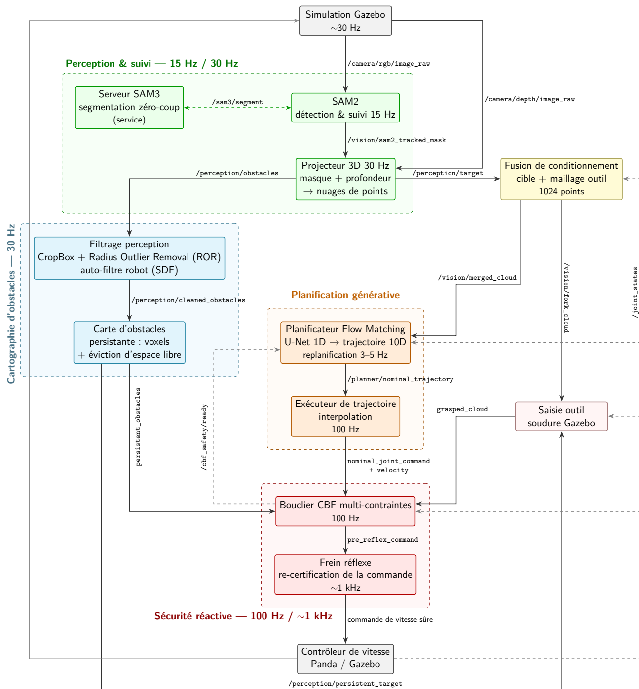
Figure 4.1 Architecture globale du système asynchrone.
