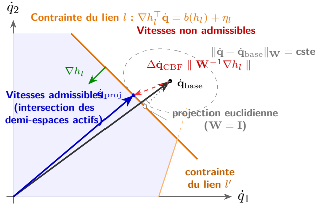
Figure 4.7 Interprétation géométrique, dans un plan de l'espace des vitesses articulaires, de la projection de sécurité (4.12) : la vitesse nominale filtrée \dot{\mathbf{q}}_{\text{base}} est projetée sur l'intersection des demi-espaces actifs \nabla h_l^\top \dot{\mathbf{q}} \geq b(h_l) + \eta_l , dont les normales \nabla h_l pointent vers l'intérieur. La solution \dot{\mathbf{q}}_{\text{proj}} est le point où le plus petit ellipsoïde de niveau de la métrique de tâche \mathbf{W} centré sur \dot{\mathbf{q}}_{\text{base}} touche la frontière : la correction \Delta \dot{\mathbf{q}}_{\text{CBF}} suit la direction \mathbf{W}^{-1} \nabla h_l et non la normale, et s'écarte ainsi de la projection euclidienne ( \mathbf{W} = \mathbf{I} , point creux), en déplaçant le moins possible le lien contrôlé.
