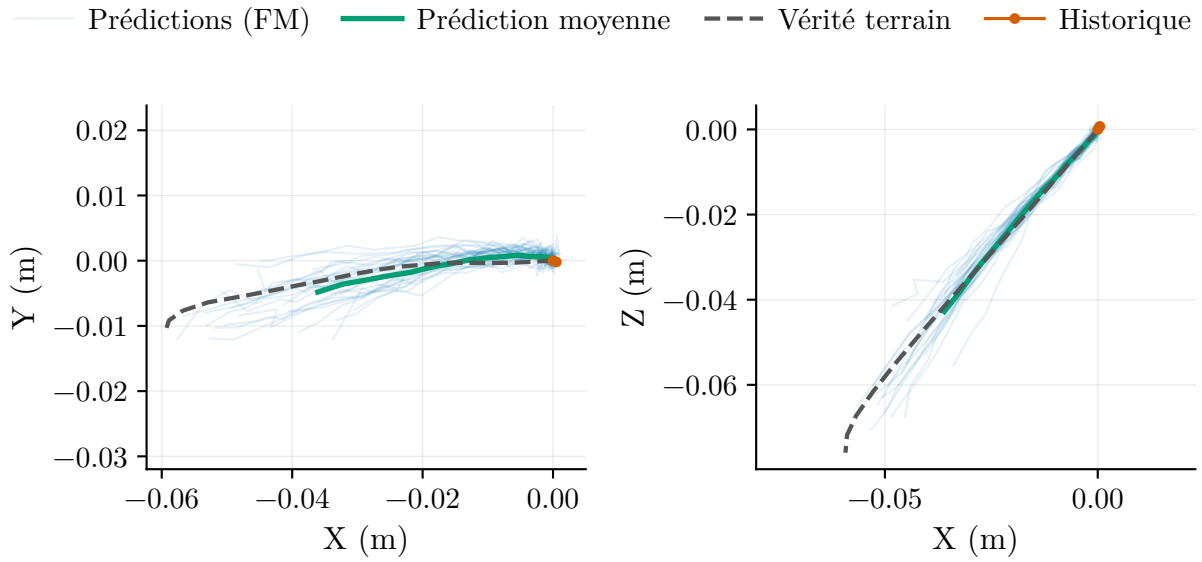
Figure I.8 Générations multiples du planificateur pour une même observation, superposées à la vérité terrain. (a) Plan XY ; (b) plan XZ .
