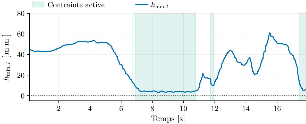
Figure 5.9 Essai représentatif de la tâche de saisie et dépôt en présence du prisme statique : évolution de la barrière h_{\min,t} . Les bandes ombrées marquent les cycles où la contrainte de sécurité évaluée sur la vitesse nominale est violée, c'est-à-dire ceux où la projection intervient.
