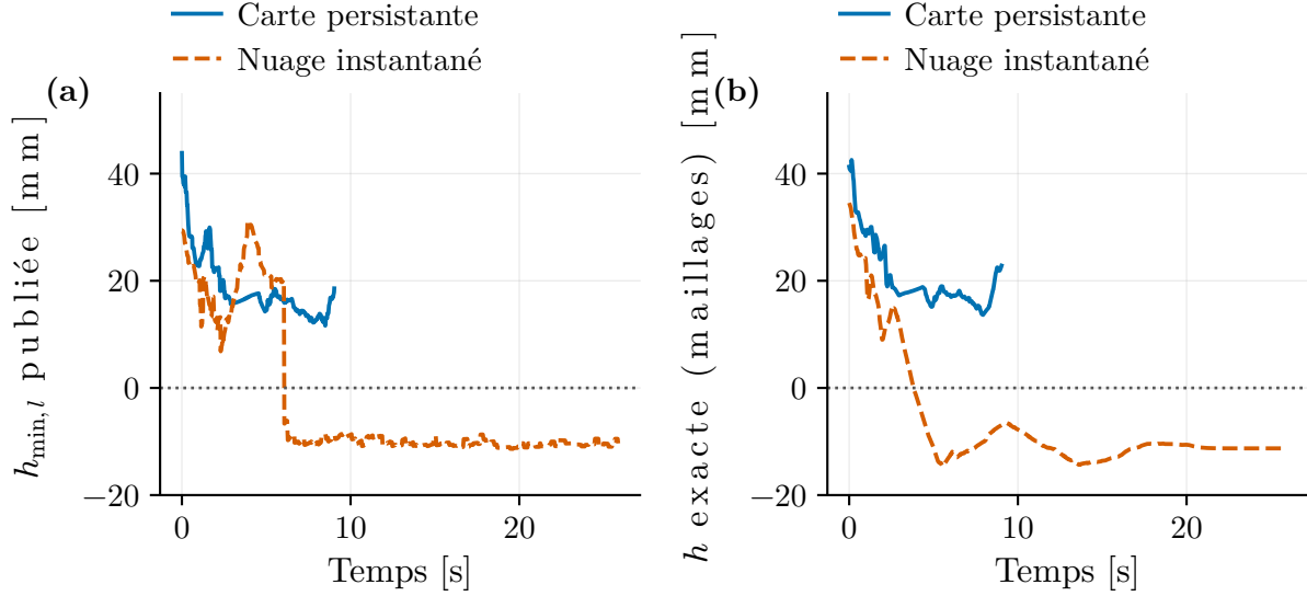
Figure 5.12 Ablation de la carte persistante sur le banc d'alimentation. (a) Barrière publiée en ligne; (b) barrière exacte recalculée hors ligne.
