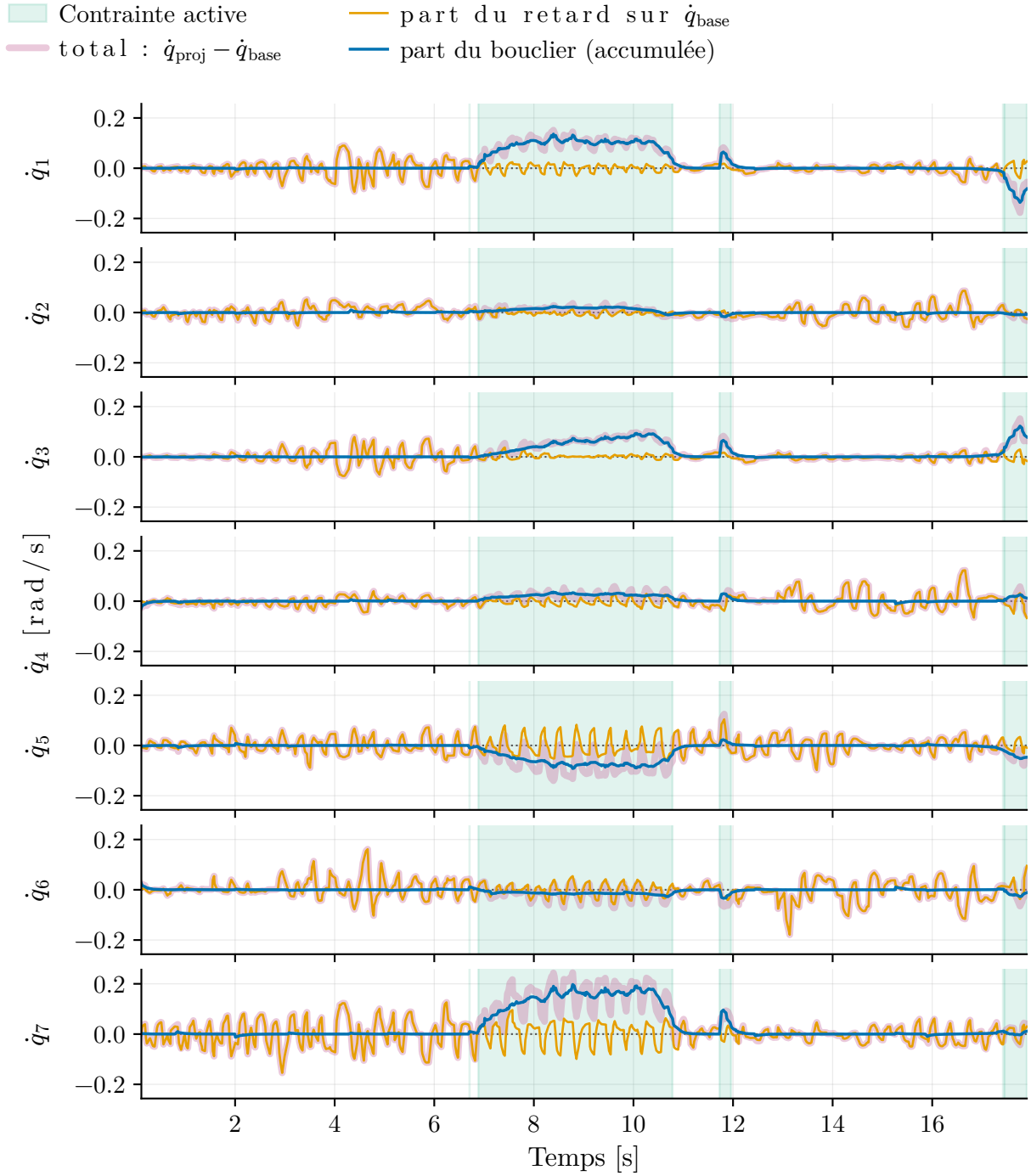
Figure 5.11 Décomposition de l'écart de la commande à la nominale, \dot{q}_{\text{proj}} - \dot{q}_{\text{base}} , pour le même essai. Les deux contributions sont celles, accumulées, de l'action du solveur et du retard du filtre sur une nominale qui varie ; séparer les incréments d'un seul cycle attribuerait au filtre la mémoire des corrections antérieures du bouclier. Les contributions étant vectorielles, elles peuvent se compenser partiellement.
