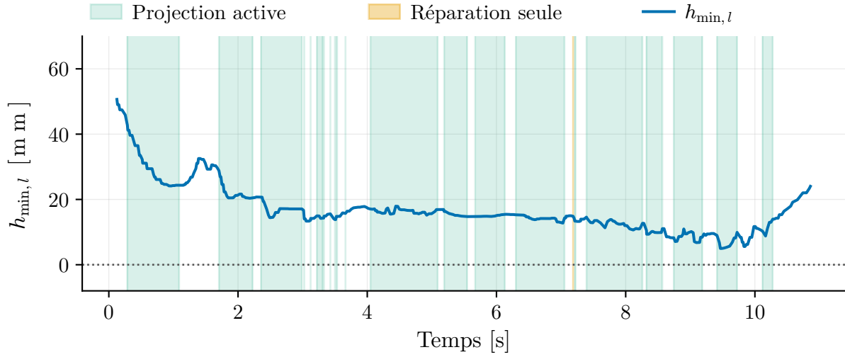
Figure 5.7 Évolution de la barrière h_{\min,l} pour une tâche en présence d'obstacles ; les bandes vertes indiquent les cycles où la projection corrige la vitesse, les bandes jaunes ceux où seule la réparation intervient.
