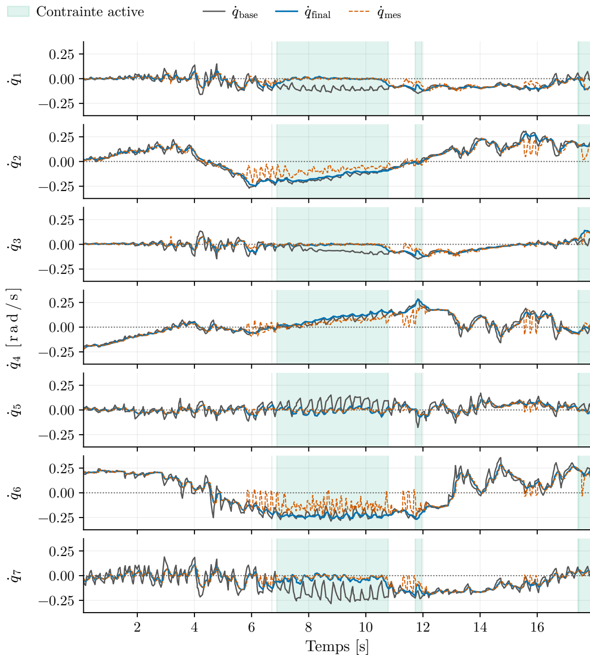
Figure 5.10 Vitesses articulaires du même essai que la Figure 5.9, relevées articulation par articulation : vitesse nominale \dot{q}_{\text{base}} , commande publiée \dot{q}_{\text{final}} et vitesse mesurée \dot{q}_{\text{mes}} . L'échelle verticale est commune aux sept articulations et les bandes ombrées sont celles de la Figure 5.9.
