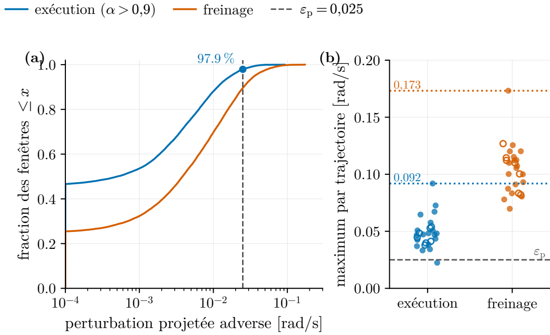
Figure 5.13 Calibration de la borne de poursuite \varepsilon_p sur 26 trajectoires de saisie et dépôt. (a) Fonction de répartition de la perturbation projetée; (b) perturbation maximale par trajectoire et bornes de prédiction non paramétriques.
