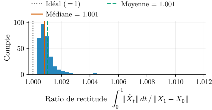
Figure I.4 Distribution du rapport de rectitude des chemins d'intégration du Rectified Flow sur le jeu de validation.
