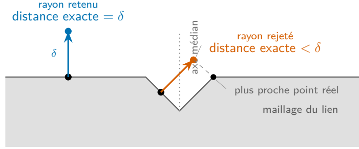
Figure D.1 Vérification des rayons normaux. À gauche, le point déplacé le long de la normale conserve son point de départ pour plus proche voisin sur le maillage : sa distance exacte vaut le décalage \delta et le rayon est retenu. À droite, la gorge fait passer le point déplacé au delà de l'axe médian : son plus proche point réel se trouve ailleurs sur le maillage, sa distance exacte est inférieure à \delta , et le rayon est rejeté. Sans cette vérification, la valeur de distance et la direction du gradient associées à ce candidat seraient erronées.
