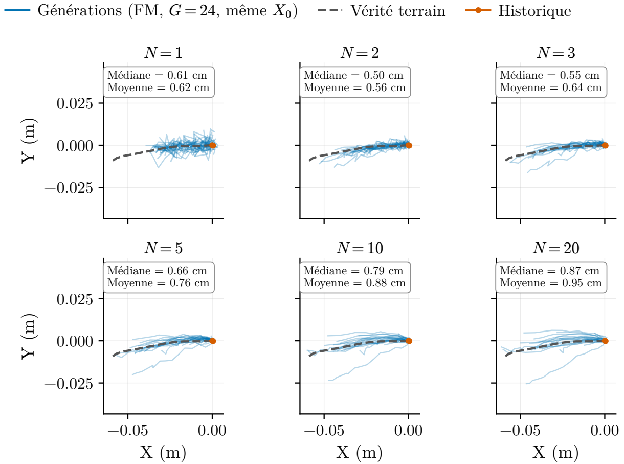
Figure I.6 Trajectoires générées dans le plan XY selon le nombre de pas d'intégration N .
