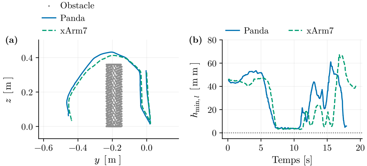
Figure 5.14 Panda et xArm7 sur un même tirage aléatoire du scénario à prisme statique. (a) Trajectoire de la pointe de l’outil dans le plan yz , superposée au nuage d’obstacles ; (b) barrière h_{\min, l} au cours de l’essai.
