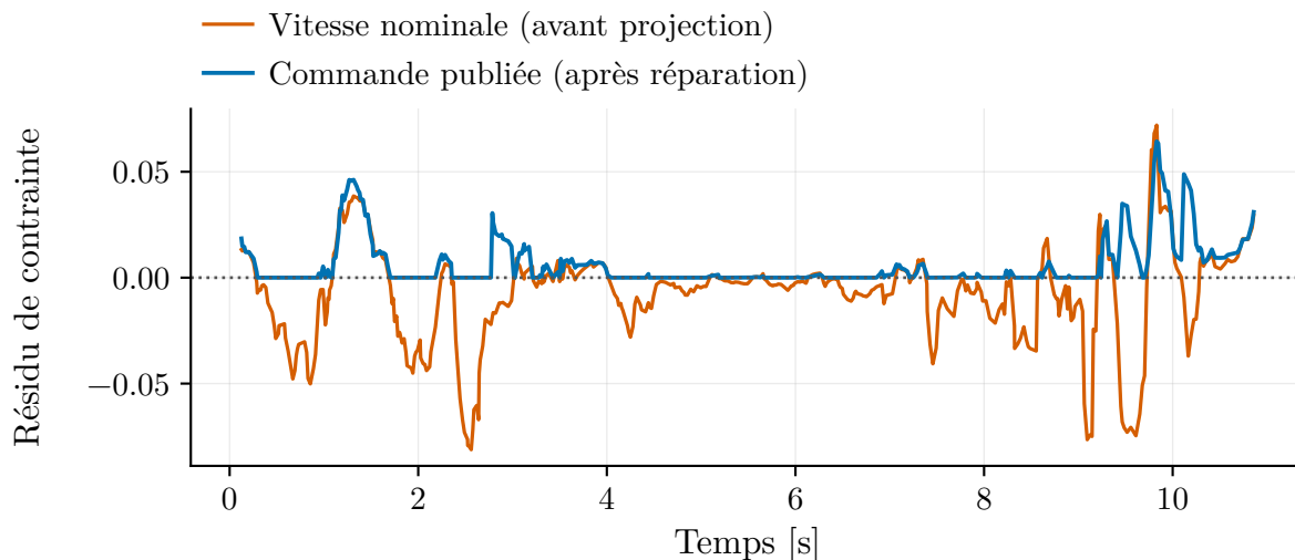
Figure 5.8 Contrainte de sécurité évaluée sur la vitesse nominale (avant projection) et sur la commande finale (après réparation). Les valeurs négatives de la courbe nominale correspondent aux violations qu'aurait commises la trajectoire générée sans filtre.
