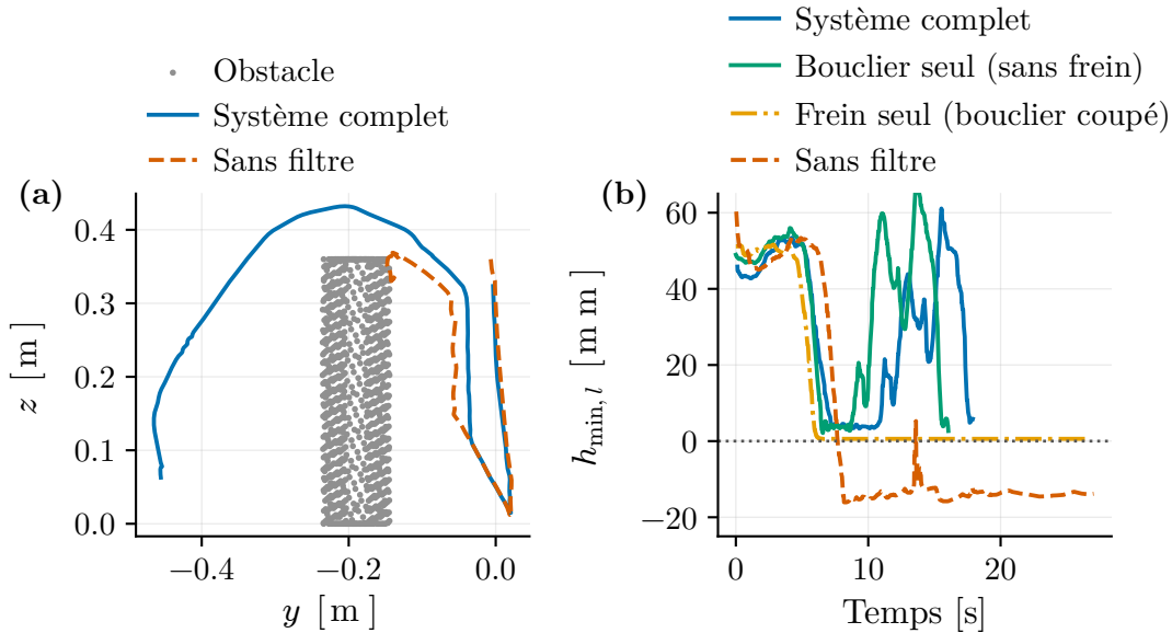
Figure 5.6 Comparaison des quatre conditions sur une même graine du banc de saisie et dépôt (prisme statique). (a) Trajectoire de la pointe de l'outil dans le plan yz , superposée au nuage d'obstacles ; (b) barrière h_{\min, l} au cours de l'essai.
