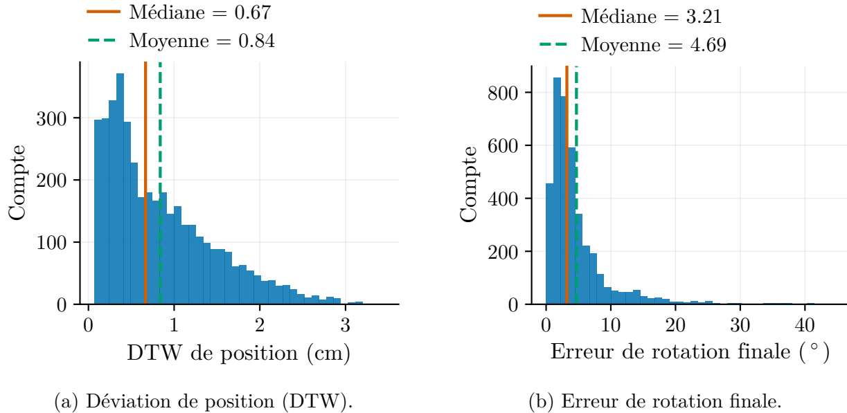
Figure I.7 Fidélité du planificateur nominal aux démonstrations expertes sur le jeu de validation. (a) Distribution de la déviation de position (DTW) ; (b) distribution de l'erreur de rotation finale à l'effecteur.
