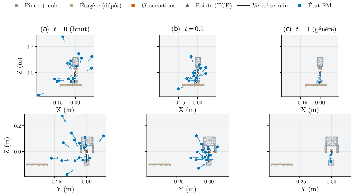
Figure I.19 Intégration du flot pour la tâche de saisie et dépôt aux instants t = 0 , t = 0,5 et t = 1 .
