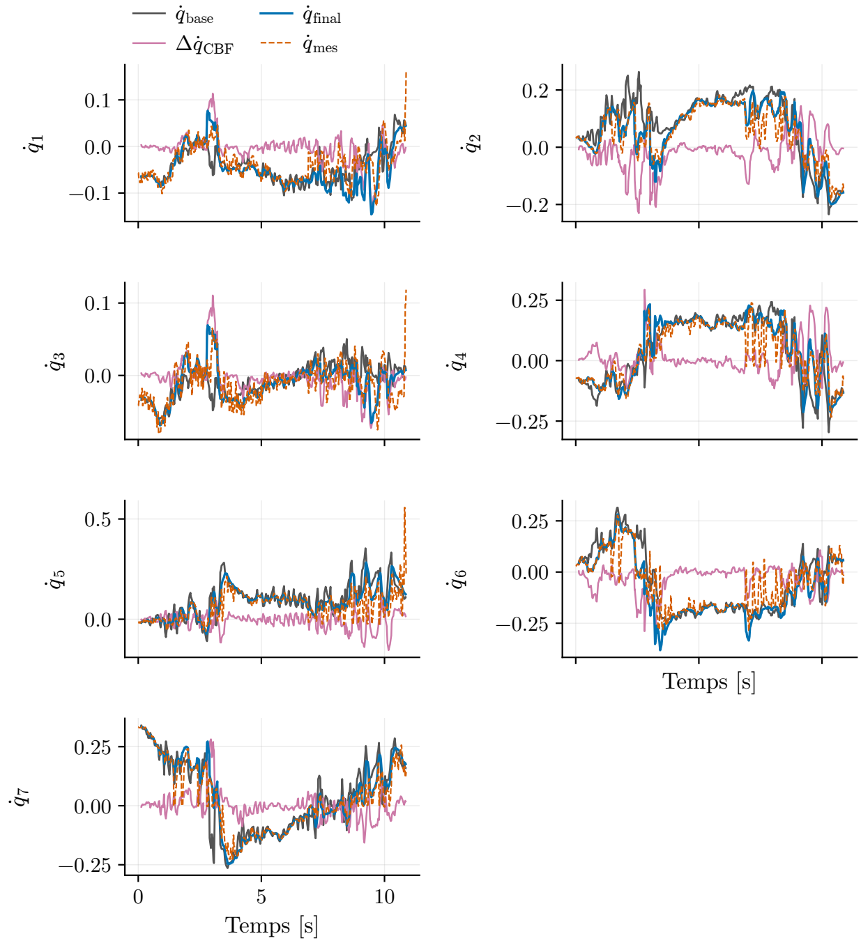
Figure I.14 Vitesse nominale, correction de projection, vitesse commandée et vitesse mesurée pour chacune des sept articulations.
