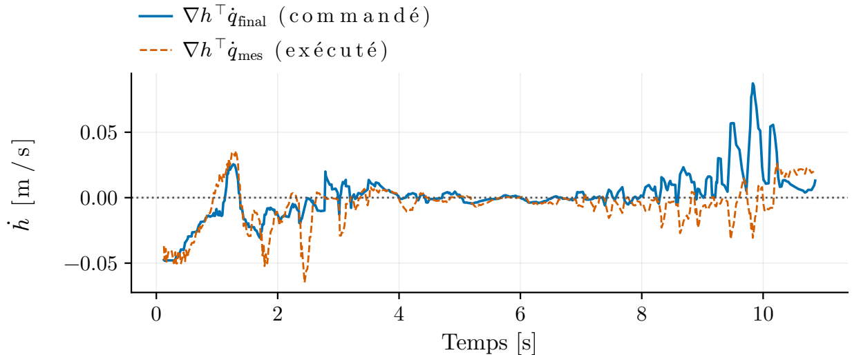
Figure I.15 Taux de variation de la barrière commandé ( \nabla h^T \dot{\mathbf{q}}_{\text{final}} ) et réellement exécuté ( \nabla h^T \dot{\mathbf{q}}_{\text{mes}} ) avec l'interface de commande retenue.
