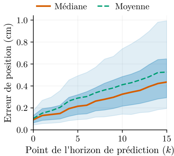
(a) Erreur de position.
