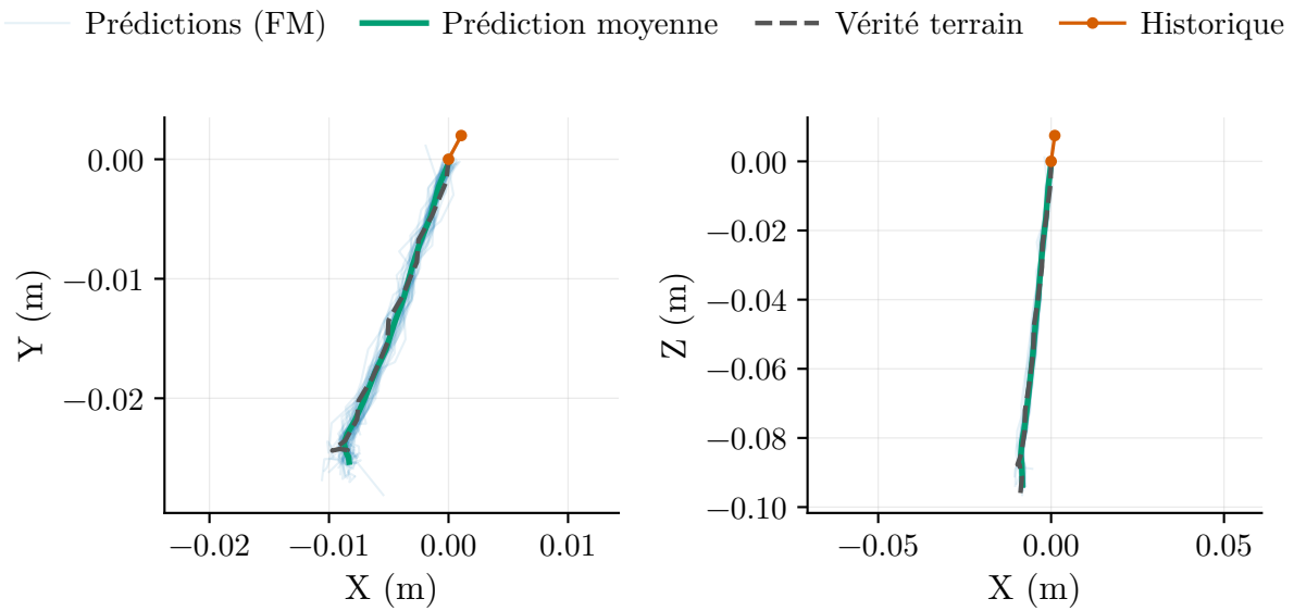
Figure I.18 Générations multiples du planificateur pour une même observation sur la tâche de saisie et dépôt, superposées à la vérité terrain.
