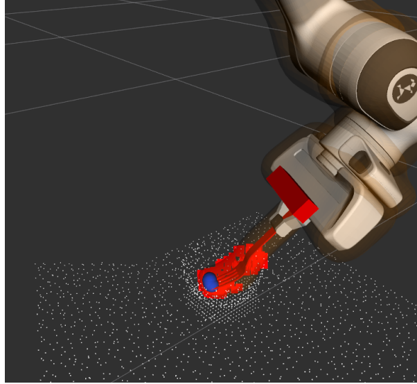
Figure I.12 Sélection des K points d'obstacles critiques et isosurface de sécurité du robot.
