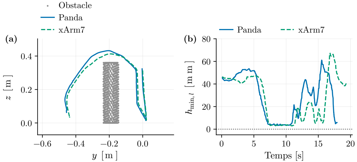
Figure 5.14 Panda et xArm7 sur une même graine du scénario à prisme statique. (a) Trajectoire de la pointe de l’outil dans le plan yz , superposée au nuage d’obstacles ; (b) barrière h_{\min, t} au cours de l’essai.
