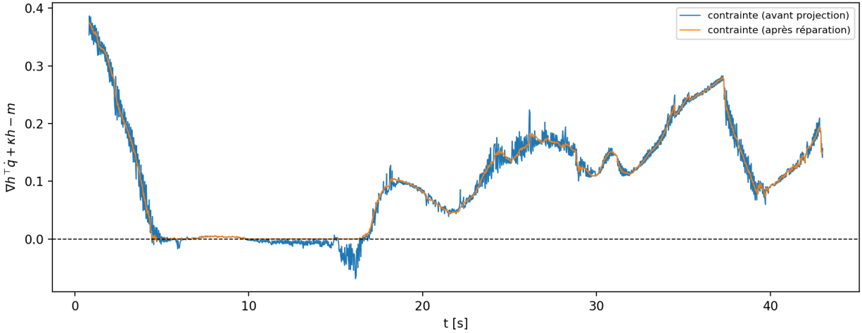
FIGURE 5.6 Évolution de la contrainte CBF pour une tâche avec présence d'obstacle
