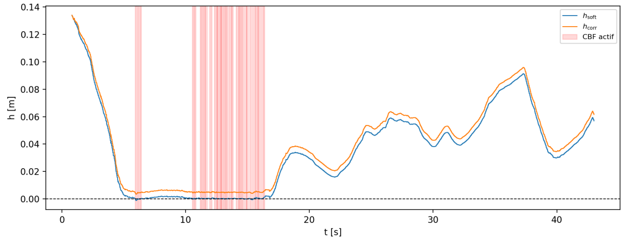
FIGURE 5.5 Évolution de h(q) pour une tâche avec présence d'obstacle
