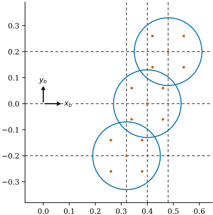
Positions d'assiette dans le repère robot (3 des 9 positions de la grille 3 \times 3 illustrées)
