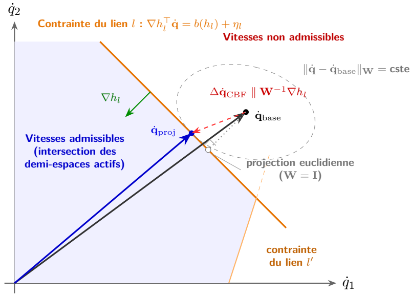
Figure 4.7 Interprétation géométrique, dans un plan de l'espace des vitesses articulaires, de la projection de sécurité (4.8) : la vitesse nominale filtrée \dot{\mathbf{q}}_{\text{base}} est projetée sur l'intersection des demi-espaces actifs \nabla h_l^\top \dot{\mathbf{q}} \geq b(h_l) + \eta_l , dont les normales \nabla h_l pointent vers l'intérieur. La solution \dot{\mathbf{q}}_{\text{proj}} est le point où le plus petit ellipsoïde de niveau de la métrique de tâche \mathbf{W} centré sur \dot{\mathbf{q}}_{\text{base}} touche la frontière : la correction \Delta \dot{\mathbf{q}}_{\text{CBF}} suit la direction \mathbf{W}^{-1} \nabla h_l et non la normale, et s'écarte ainsi de la projection euclidienne ( \mathbf{W} = \mathbf{I} , point creux), en déplaçant le moins possible le lien contrôlé.
