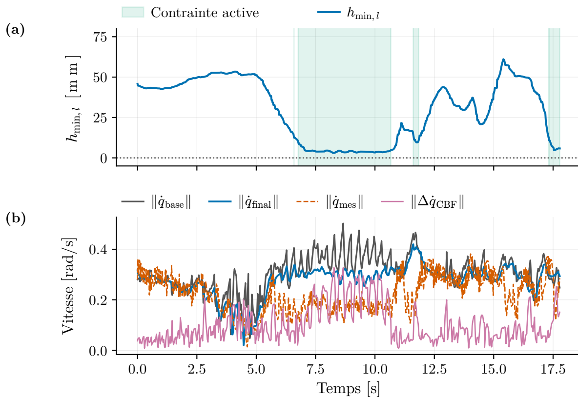
Figure 5.8 Essai représentatif de la tâche de saisie et dépôt en présence du prisme statique. (a) Barrière h_{\min, l} , les bandes ombrées marquant les cycles où la vitesse nominale ne satisfait pas la contrainte resserrée ; (b) norme de la vitesse nominale filtrée, de la commande publiée, de la vitesse articulaire mesurée et de la correction de projection.
