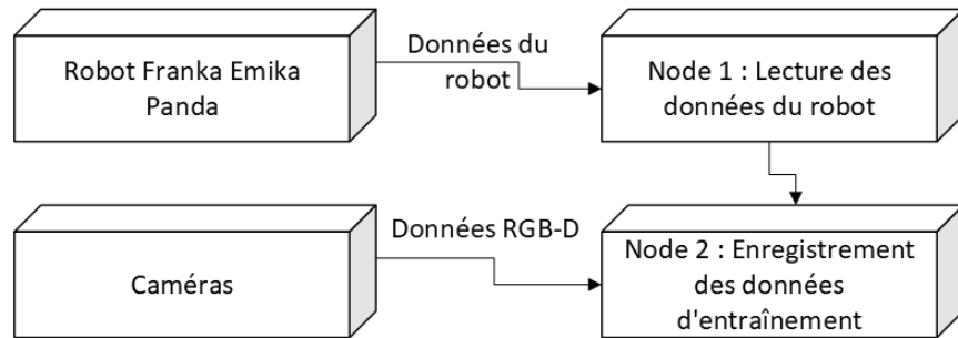
Figure 4.2 Architecture du système d'acquisition de données
