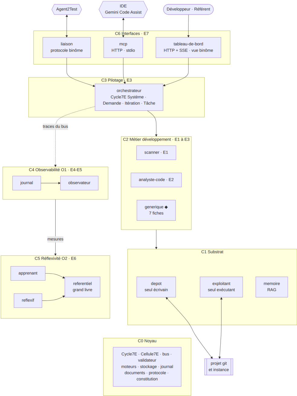
Figure 8 — Agent2Dev, architecture §3.1 Diagramme de composants (UML, en flowchart Mermaid) — couches et modules
