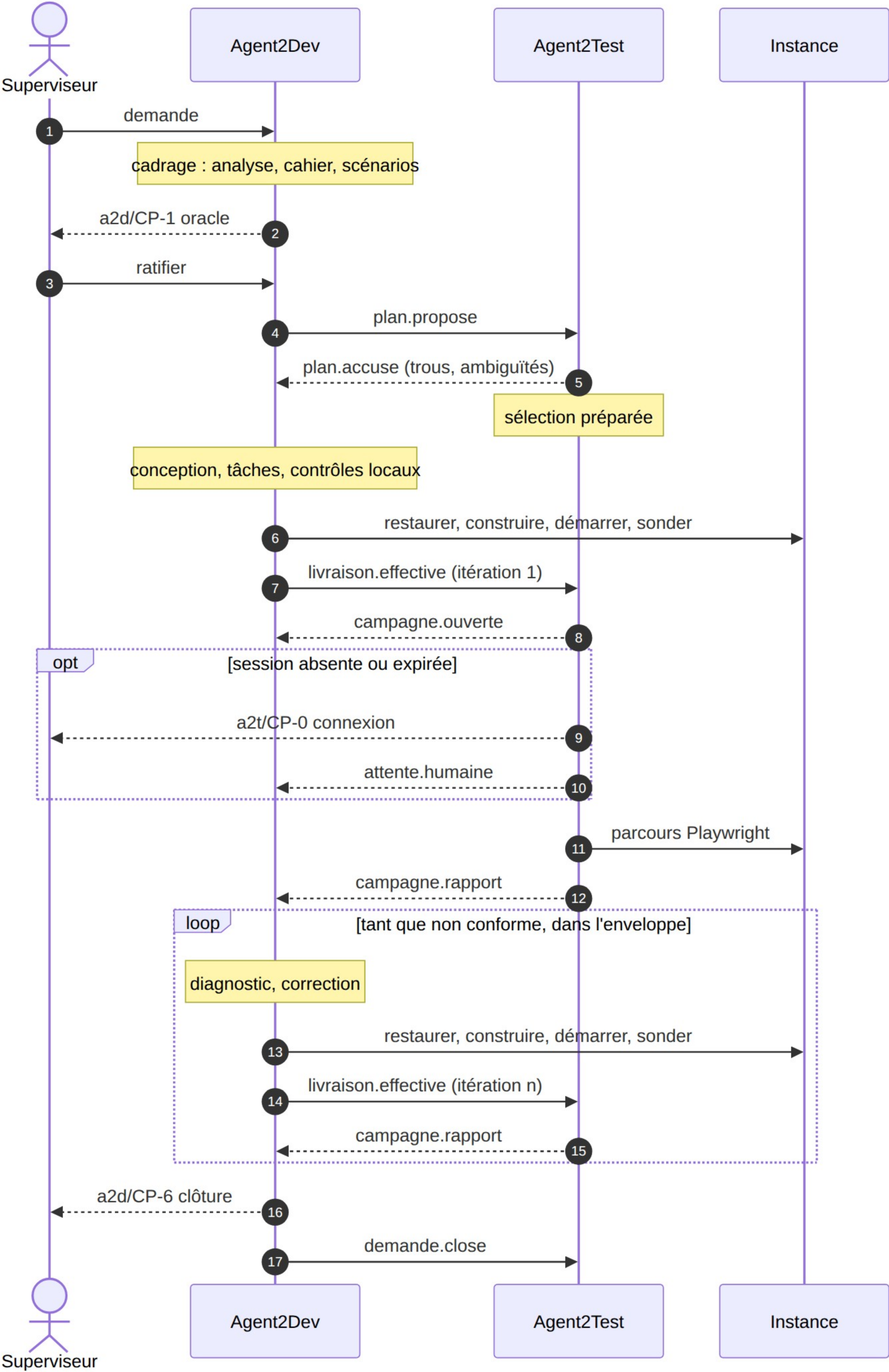
Figure 4 — Binôme §4.4 — Diagramme de séquence
