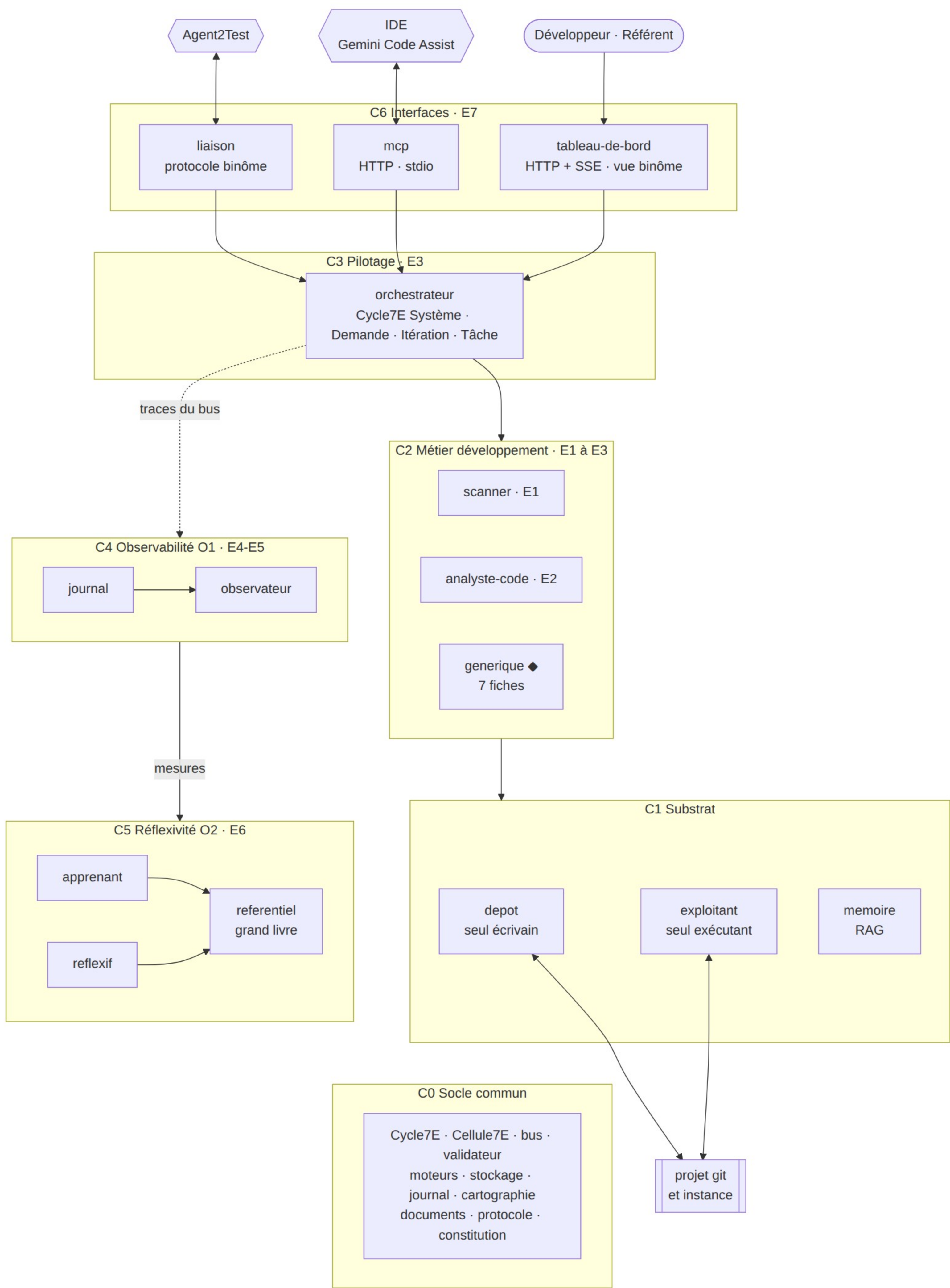
Figure 8 — Agent2Dev §3.1 — Diagramme de composants — couches et modules
