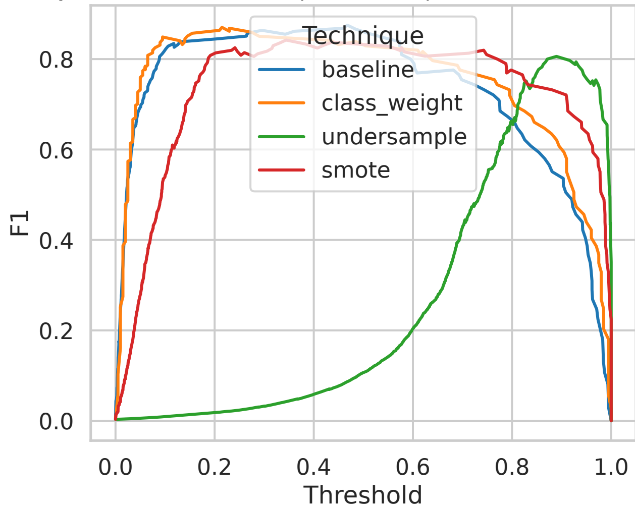
RQ1: Threshold vs F1 (validation) – RandomForest (CC)
